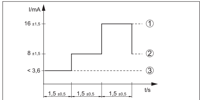
Fig. 12: Diagrama de operaciones del control de funcionamiento (Modo de operación "max")
