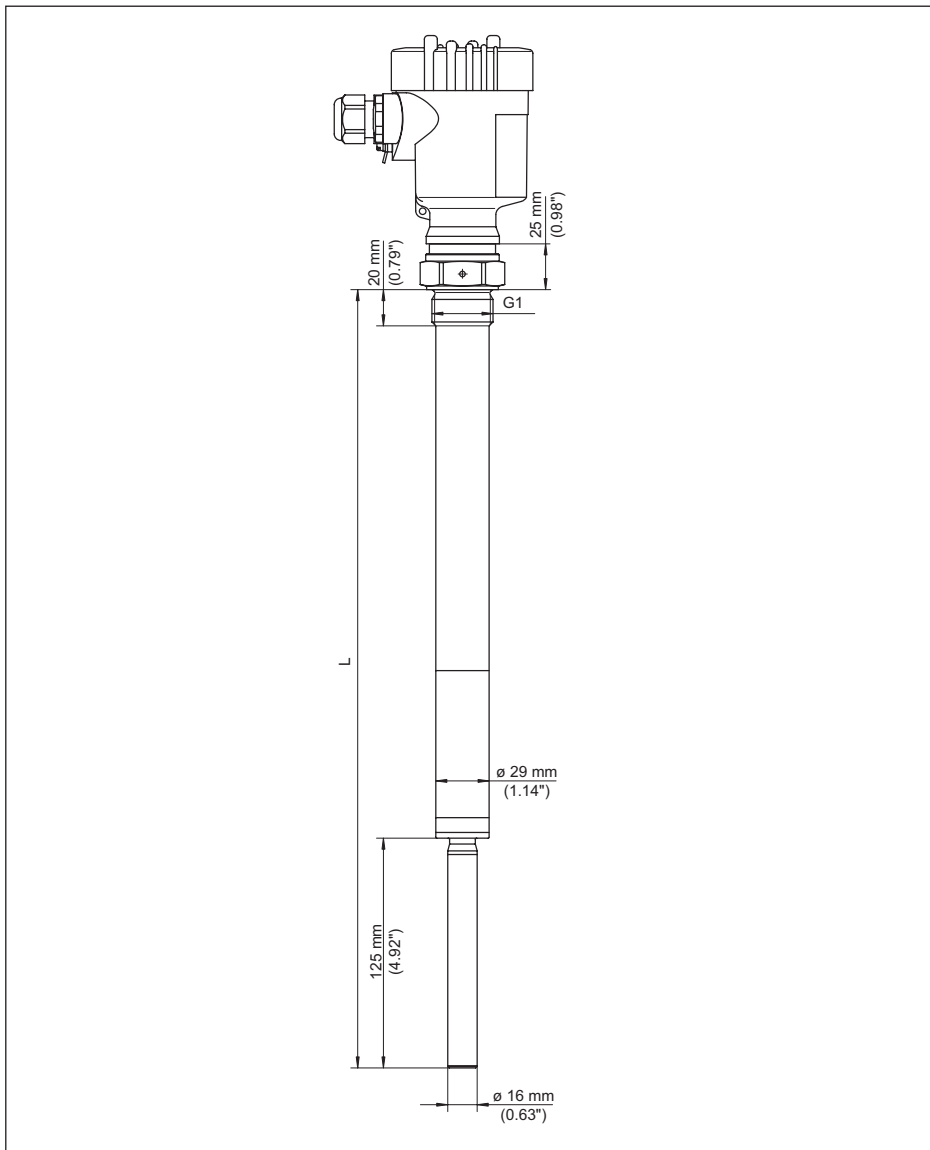
Fig. 18: VEGAVIB 63, versión roscada G1 (DIN ISO 228/1)
