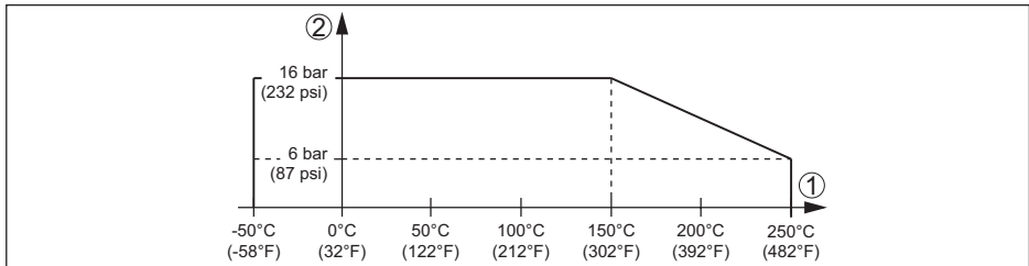
Fig. 14: Presión de proceso - temperatura de proceso
