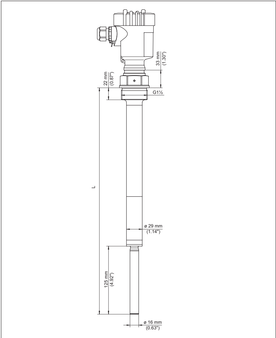
Fig. 19: VEGAVIB 63, versión roscada G1½ (DIN ISO 228/1)
