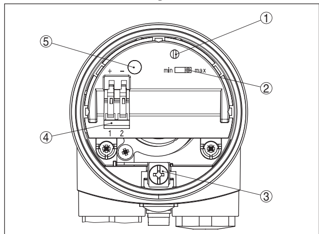
Fig. 11: Compartimento de la electrónica y de conexiones - Salida de dos hilos
