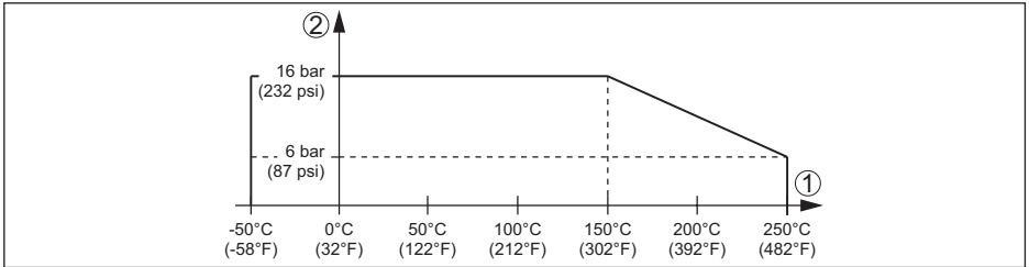
Res. 14: Proses basıncı - Proses sıcaklığı
