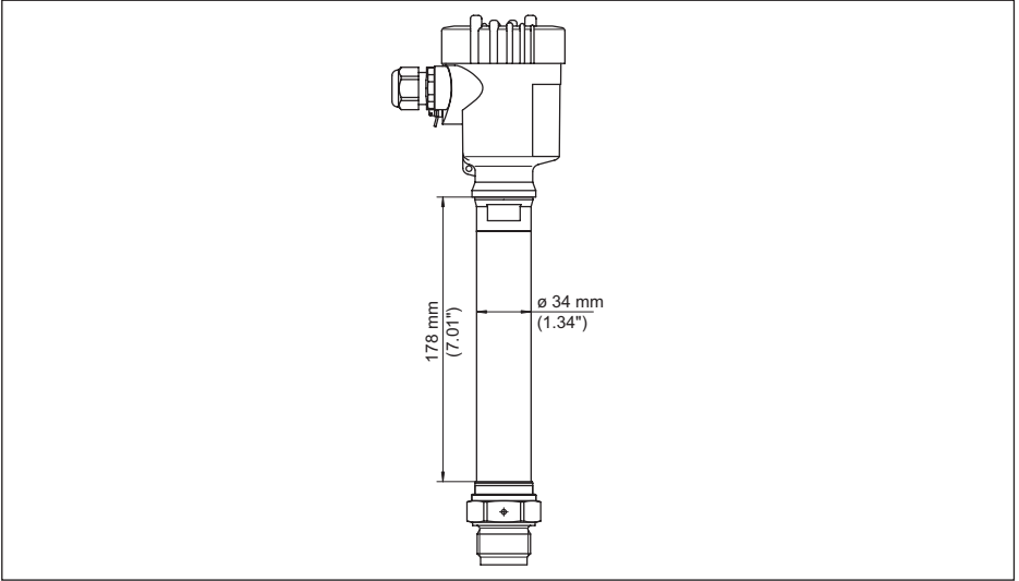
Res. 20: Sıcaklık adaptörü
