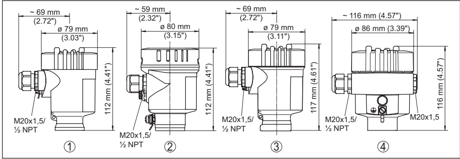
Res. 16: IP66/IP67 ve IP66/IP68 koruma tipinde gövde modelleri; 0,2 bar
