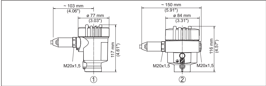
Res. 17: IP66/IP68 koruma tipinde gövde modelleri (1 bar)
