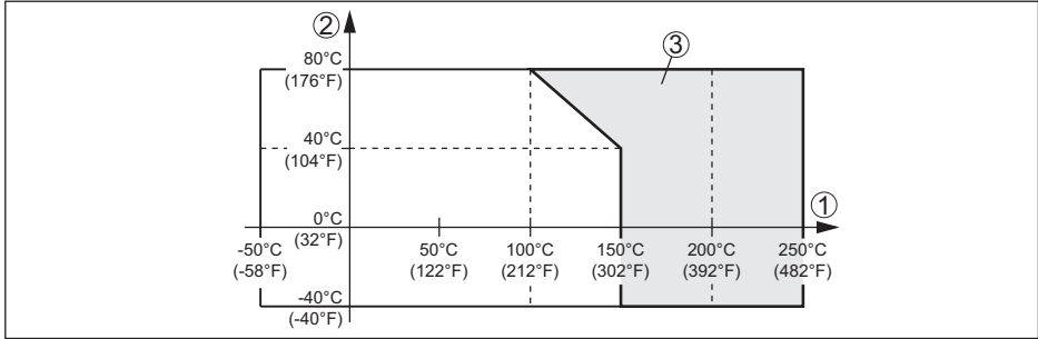
Res. 15: Ortamdaki maddenin sıcaklığı - Proses sıcaklığı
