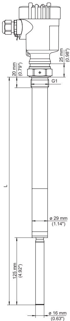
Fig. 15: VEGA VIB 63, Modelo com rosca G1 (DIN ISO 228/1)
