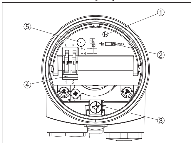
Fig. 10: Compartimento do sistema eletrônico e de conexão - interruptor sem contato
