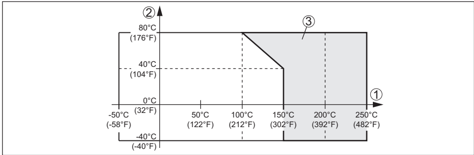
Fig. 17: Temperatura ambiente - Temperatura de proceso
