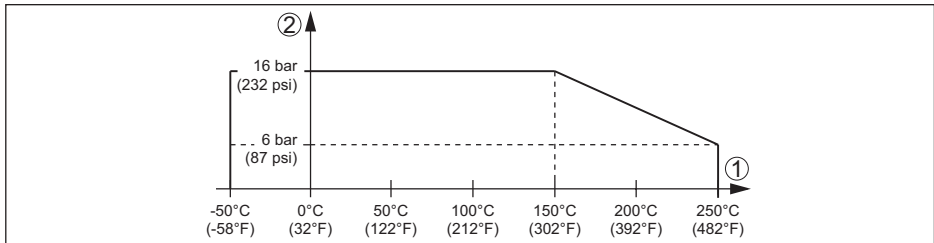
Fig. 16: Presión de proceso - temperatura de proceso
