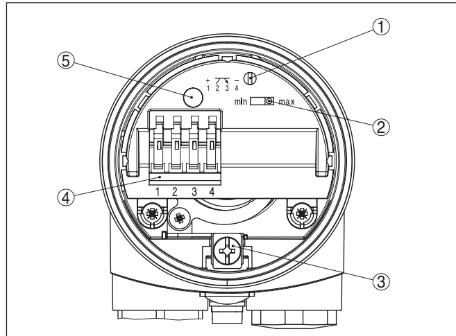
Fig. 14: Compartiment électronique et de raccordement - sortie transistor
