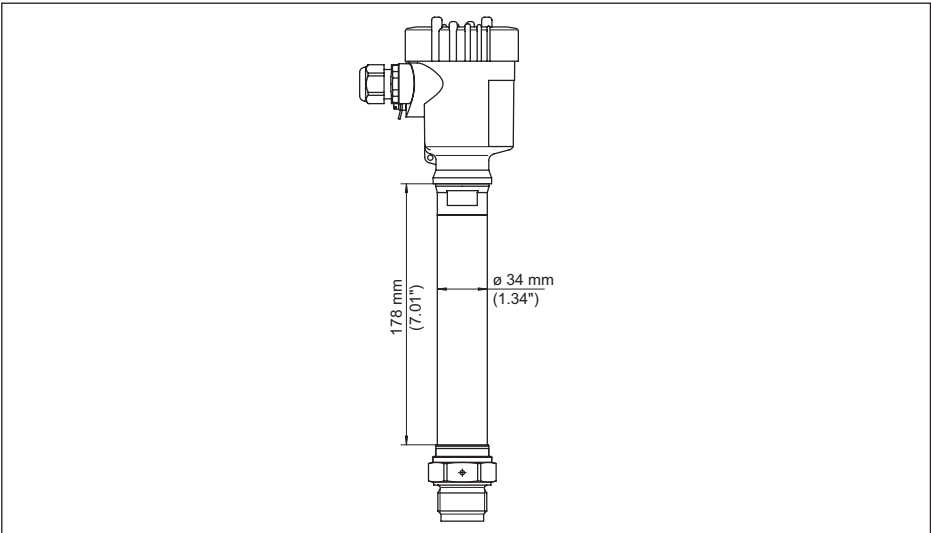
Fig. 22: Extension haute température
