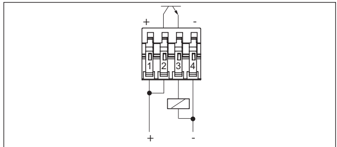
Fig. 12: Comportement PNP
