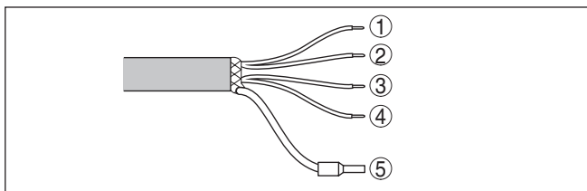
Fig. 13: Affectation des conducteurs du câble de raccordement. Les numéros des conducteurs correspondent aux bornes de raccordement de l'appareil.
