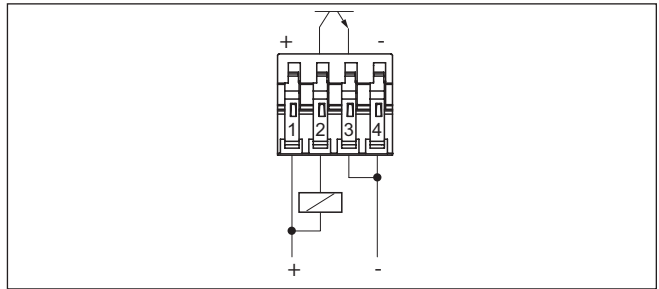
Fig. 11: Comportement NPN
