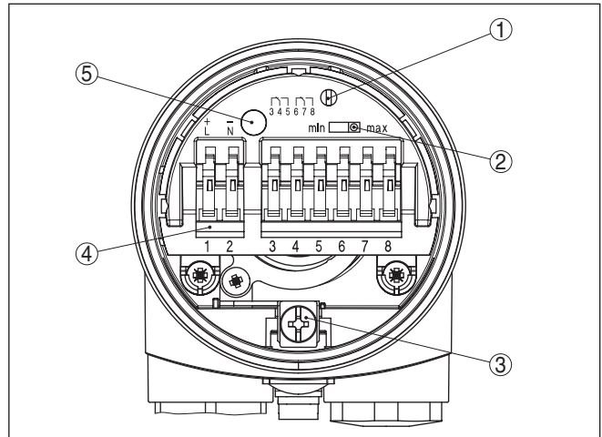
Fig. 11: Compartimento do sistema eletrônico e de conexão - Saída de relé
