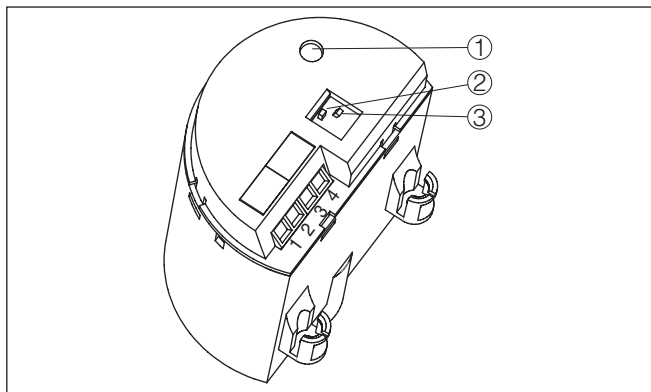
Figura 14: Unità elettronica SWE60T - Uscita a transistor
