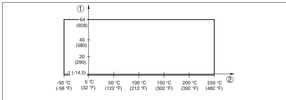
Figura 19: Temperatura di processo - Pressione di processo con posizione del commutatore \geq 0,7 \text{ g/cm}^3 (commutatore di sensibilità)
