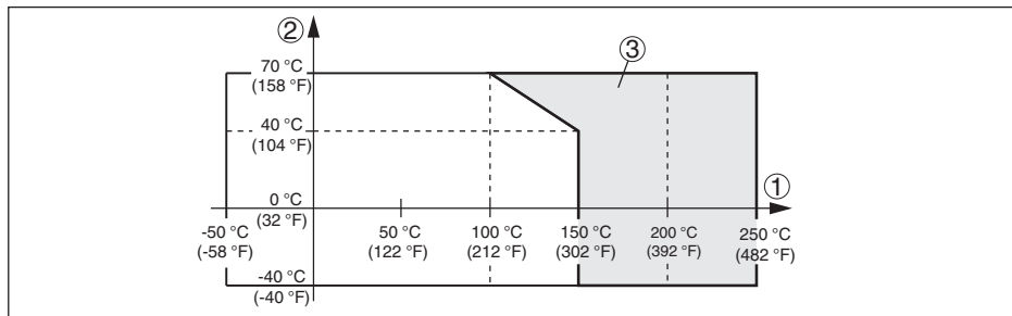
Figura 18: Temperatura ambiente - Temperatura di processo
