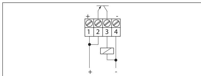
Figura 12: Comportamento PNP
