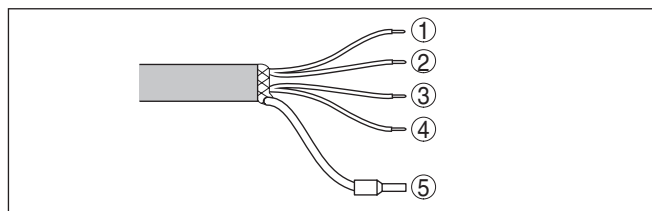
Figura 13: Numerazione dei conduttori del cavo di collegamento. I numeri dei conduttori corrispondono ai morsetti dell'apparecchio.
