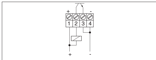
Figura 11: Comportamento NPN
