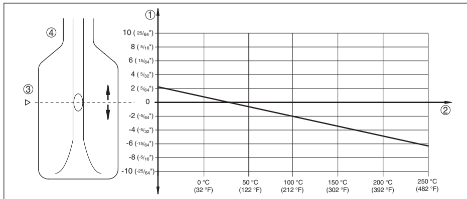
Figura 15: Influenza della temperatura di processo sul punto d'intervento
