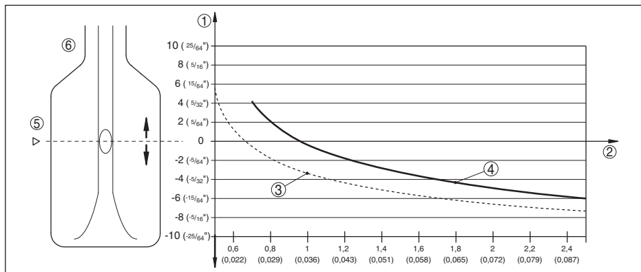
Figura 16: Influenza della densità del prodotto sul punto d'intervento
