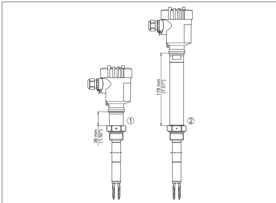
Figura 24: Opzioni
