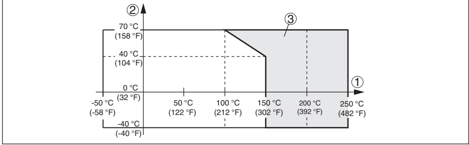
Res. 16: Ortamdaki maddenin sıcaklığı - Proses sıcaklığı
