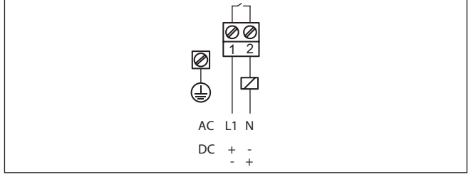
Res. 11: Bir hücreli gövdenin bağlantı şeması
