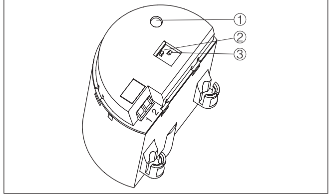
Res. 12: SWE60C Elektronik modül - Kontaklız şalter
