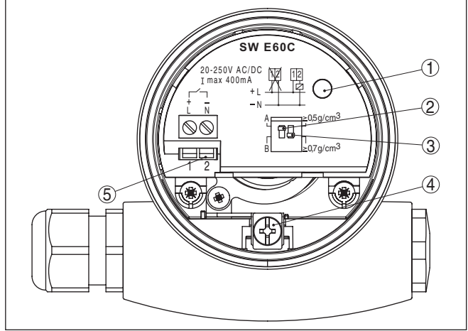
Res. 10: Bir hücreli gövdede elektronik ve bağlantı bölgesi
