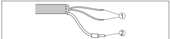
Abb. 10: Aderbelegung Anschlusskabel
