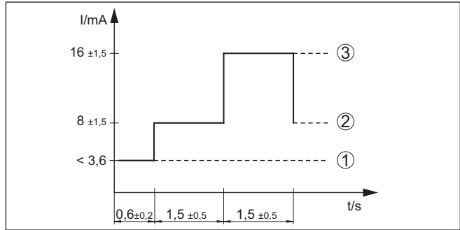
Abb. 12: Ablaufdiagramm des Funktionstests
