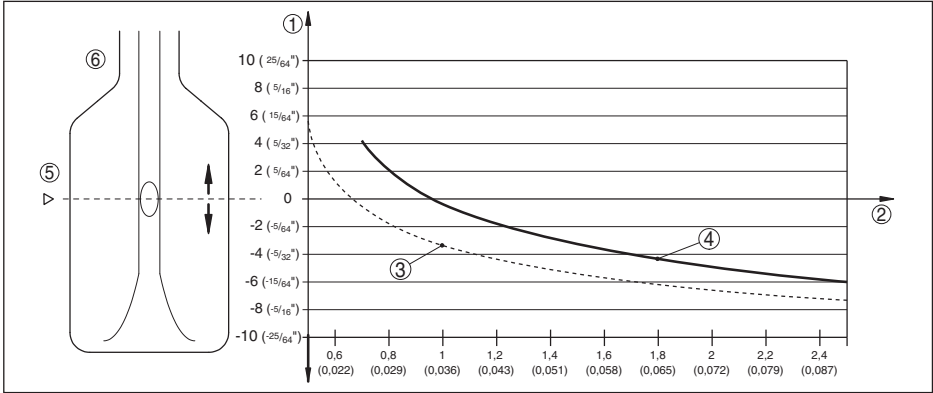
Abb. 14: Einfluss der Füllgütdichte auf den Schaltpunkt
