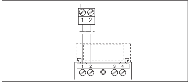
Abb. 9: Anschlussplan Einkammergehäuse
