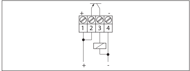
Abb. 10: PNP-Verhalten
