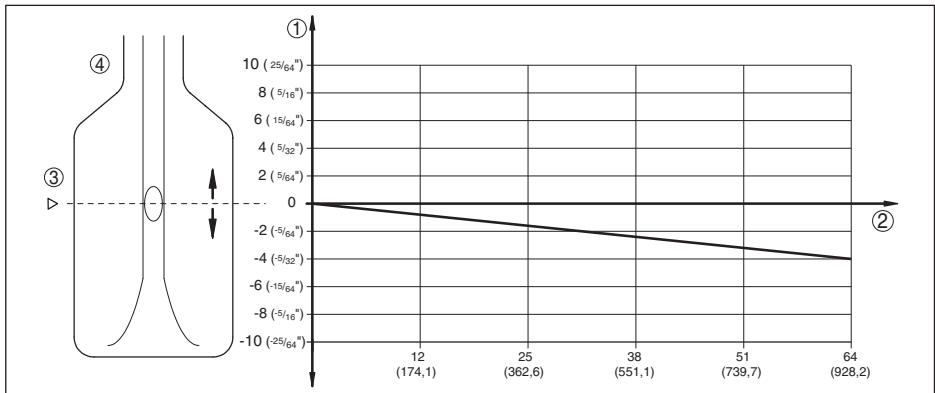
Abb. 15: Einfluss des Prozessdruckes auf den Schaltpunkt
