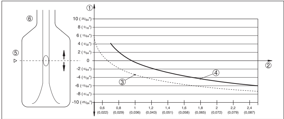
Abb. 14: Einfluss der Füllgutedichte auf den Schaltpunkt
