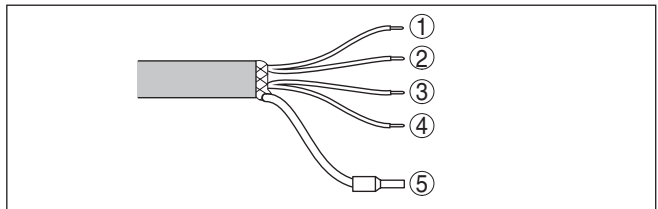
Abb. 11: Aderbelegung Anschlusskabel. Die Nummern der Adern entsprechen den Anschlussklemmen des Gerätes.
