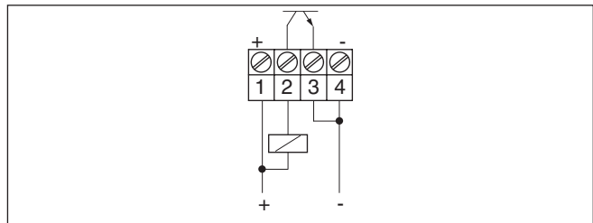
Abb. 9: NPN-Verhalten
