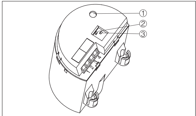
Abb. 12: Elektronikereinsatz SWE60T - Transistorausgang
