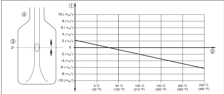
Abb. 13: Einfluss der Prozesstemperatur auf den Schaltpunkt
