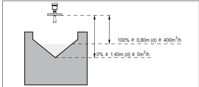
Figura 14: Taratura di misura di portata con stramazzo triangolare
