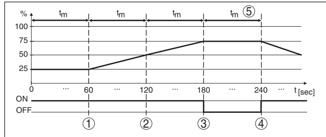
Fig. 13: Exemple d'une reconnaissance de tendance
