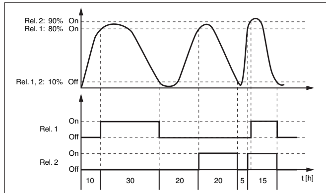
Fig. 12: Exemple pour la commande de pompes 2
