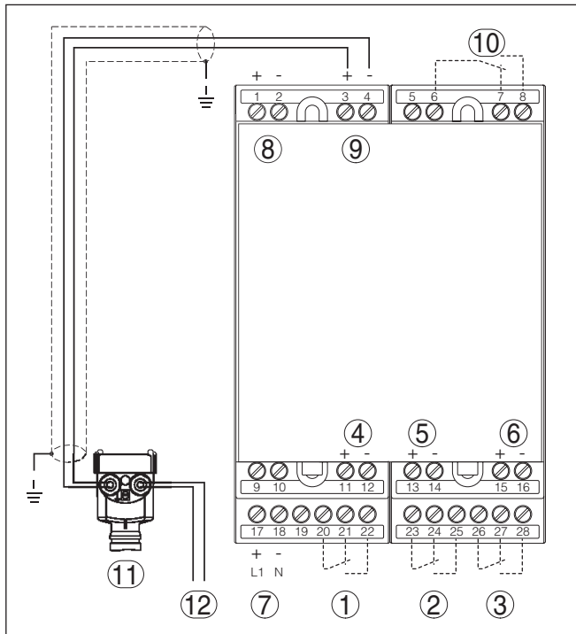
Fig. 4: Schéma de raccordement VEGAMET 624 avec capteurs 4 fils
