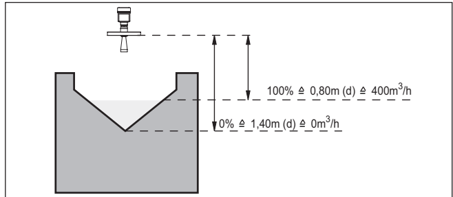
Fig. 14: Réglage de la mesure de débit dans un déversoir triangulaire
