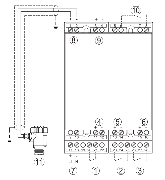
Fig. 3: Schéma de raccordement VEGAMET 624 avec capteur bifilaire
