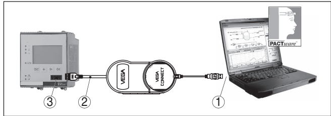
Abb. 6: Anschluss via VEGACONNECT
