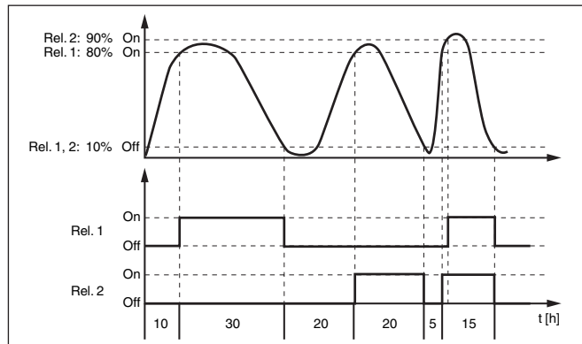
Abb. 12: Beispiel für Pumpensteuerung 2
