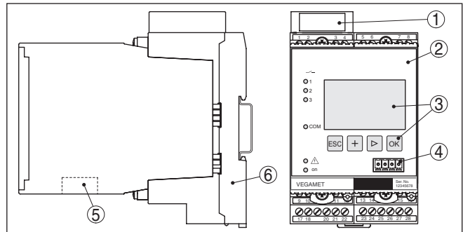
Abb. 1: VEGAMET 624
