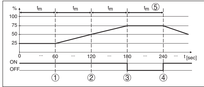
Abb. 13: Beispiel für Tendenzerkennung
