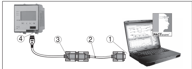
Abb. 9: Anschluss des PCs via RS232
