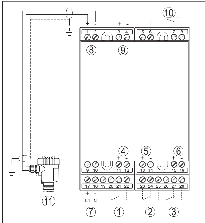
Abb. 3: Anschlussplan VEGAMET 624 mit Zweileitersensor
