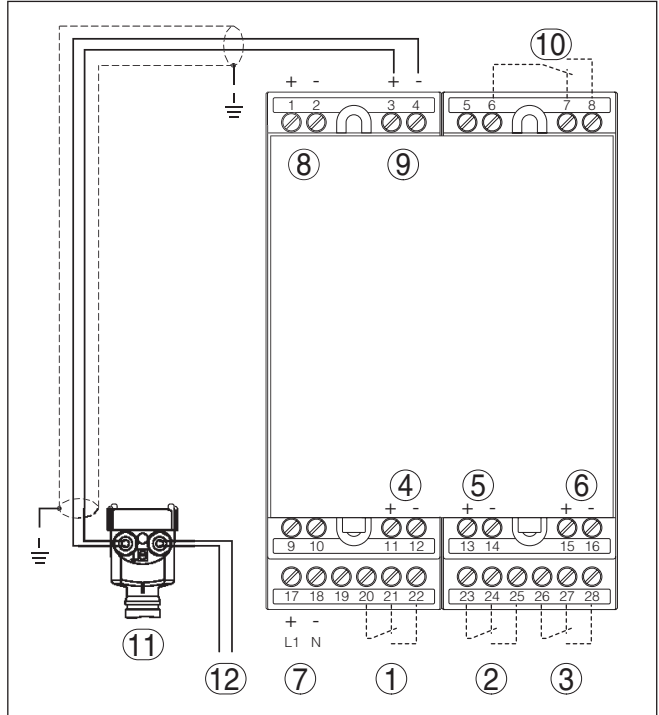
Abb. 4: Anschlussplan VEGAMET 624 mit Vierleitersensoren
