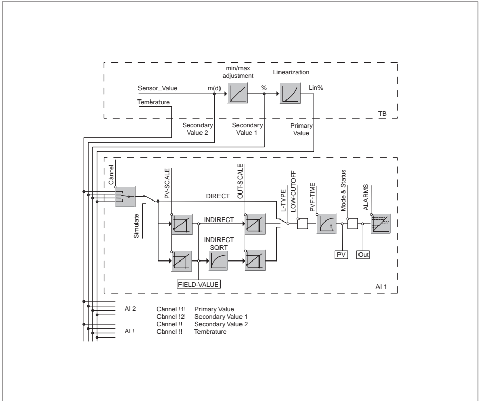
Figura 35: Elaborazione valore di misura VEGASON 62
