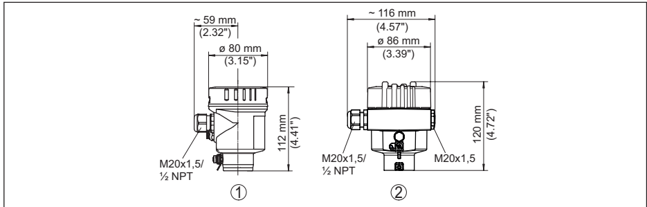
Figura 40: Differenti custodie con grado di protezione IP66/IP68 (0,2 bar), (con tastierino di taratura con display incorporato l'altezza della custodia aumenta di 18 mm/0.71 in)
