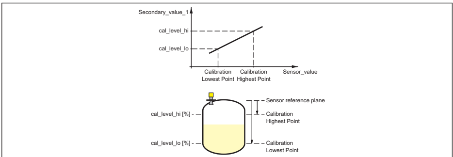
Figura 36: Taratura VEGASON 62
