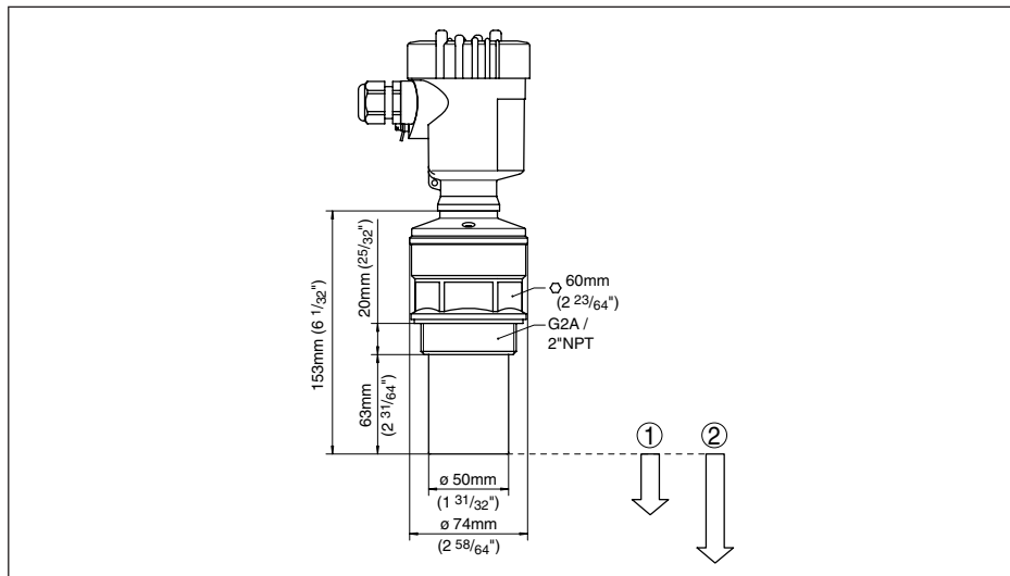
Figura 42: VEGASON 62
