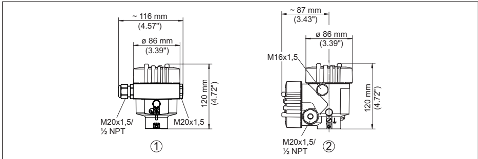
Fig. 40: Variantes de carcasa con tipo de protección IP66/IP68 (0,2 bar), (con el módulo de visualización y configuración montado aumenta la altura de la carcasa en 18 mm/0,71 in)
