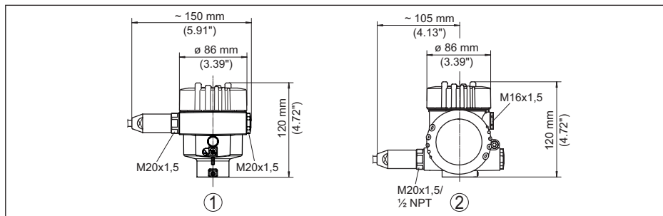
Fig. 41: Variantes de carcasa con tipo de protección IP66/IP68 (1 bar), (con el módulo de visualización y configuración montado aumenta la altura de la carcasa en 18 mm/0.71 in)
