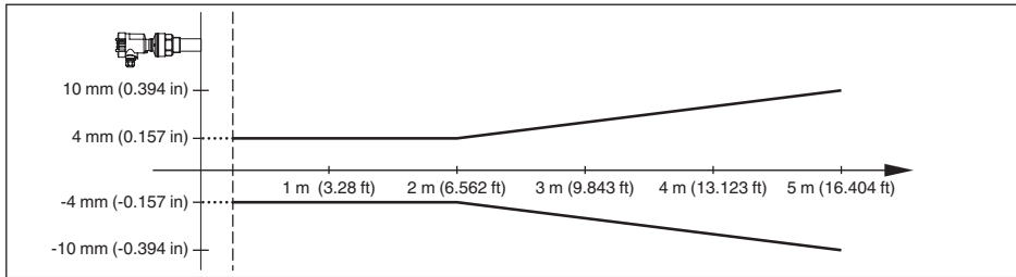
Fig. 35: Error de medición VEGASON 61
