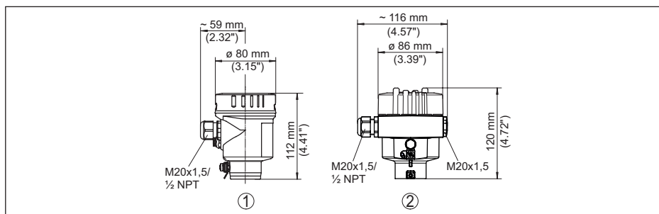
Fig. 42: Variantes de carcasa con tipo de protección IP66/IP68 (0,2 bar), (con el módulo de visualización y configuración montado aumenta la altura de la carcasa en 18 mm/0.71 in)
