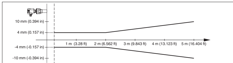
Fig. 34: Error de medición VEGASON 61
