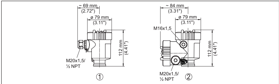
Fig. 39: Variantes de carcasa en grado de protección IP66/IP67; 1 bar (con módulo de visualización y configuración integrado aumenta la altura de la carcasa en 9 mm/0,35 in)
