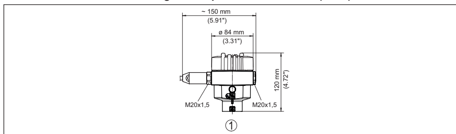
Fig. 43: Variantes de carcasa con tipo de protección IP66/IP68 (1 bar), (con el módulo de visualización y configuración montado aumenta la altura de la carcasa en 18 mm/0.71 in)
