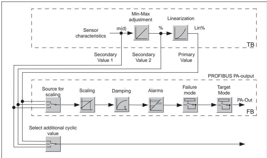
Fig. 36: VEGASON 61: Diagrama de conexión con valor AI (PA-OUT) y valor cíclico adicional
