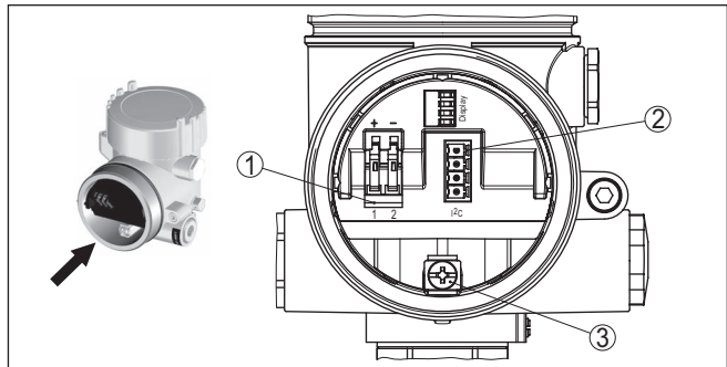
Fig. 24: Aansluitruimte - tweekamerbehuizing
