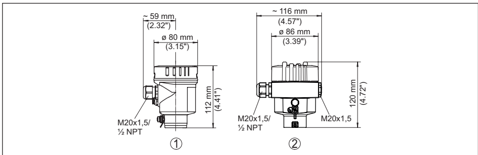
Fig. 42: Huisuitvoeringen in beschermingsklasse IP66/IP68 (0,2 bar), (met ingebouwde display- en bedieningsmodule wordt het huis 18 mm hoger)
