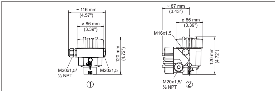
Fig. 40: Huisuitvoeringen in beschermingsklasse IP66/IP68 (0,2 bar), (met ingebouwde display- en bedieningsmodule wordt het huis 18 mm hoger)
