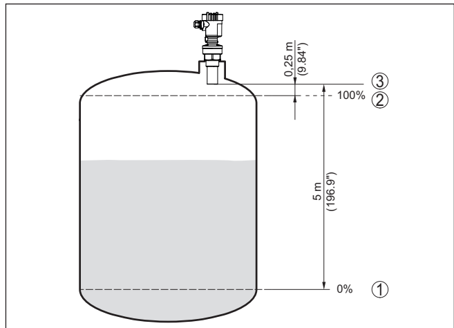
Fig. 29: Parametreervoorbeeld min.-/max.-inregeling
