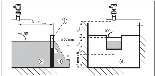
Fig. 16: Flowmeting met rechthoekig overstortschot: d_{\min} = blokafstand van de sensor (zie hoofdstuk "Technische gegevens"); h_{\max} = max. vullhoogte rechthoekige overstortschot
