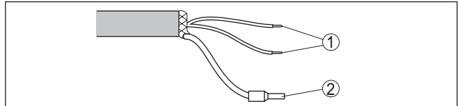
Fig. 26: Aderbezetting aansluitkabel
