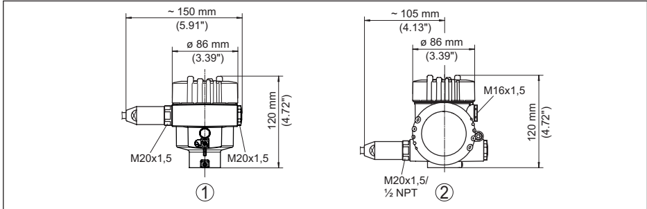
Fig. 41: Huisuitvoeringen in beschermingsklasse IP66/IP68 (1 bar), (met ingebouwde display- en bedieningsmodule wordt het huis 18 mm/0.71 in hoger)
