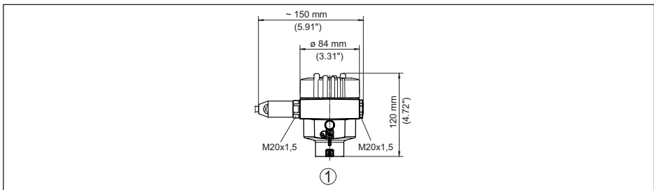
Fig. 43: Huisuitvoeringen in beschermingsklasse IP66/IP68 (1 bar), (met ingebouwde display- en bedieningsmodule wordt het huis 18 mm/0.71 in hoger)
