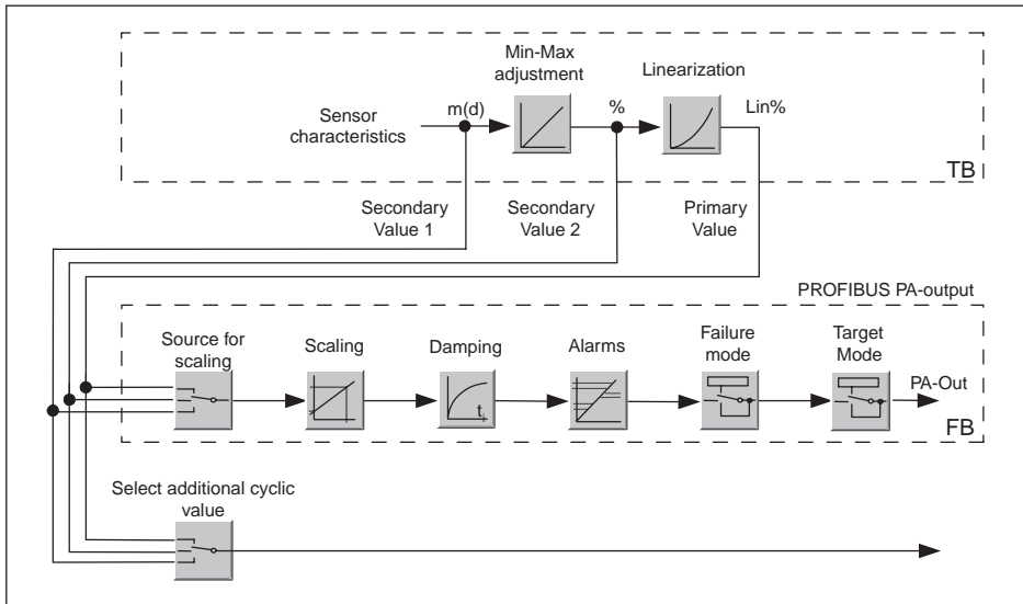
Fig. 36: VEGASON 61: blokschema met AI (PA-OUT)-waarde en extra cyclische waarde
