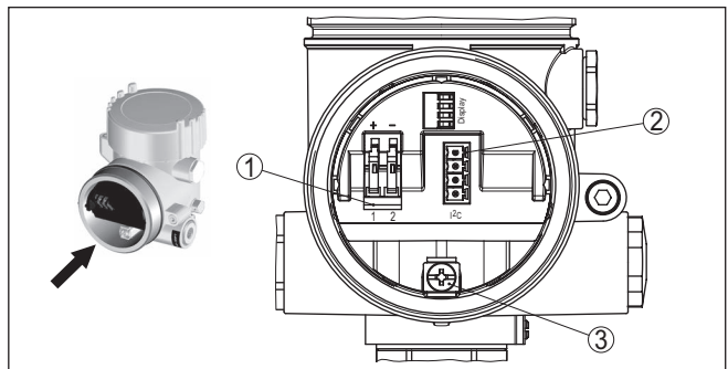
Abb. 26: Anschlussraum - Zweikammergehäuse
