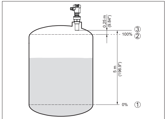
Abb. 31: Parametrierbeispiel Min.-/Max.-Abgleich
