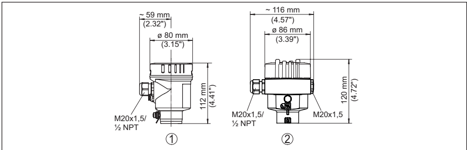
Abb. 40: Gehäuseausführungen in Schutzart IP66/IP68 (0,2 bar), (mit eingebautem Anzeige- und Bedienmodul vergrößert sich die Gehäusehöhe um 18 mm/0.71 in)
