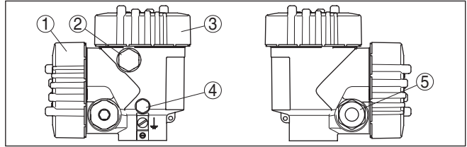
Abb. 24: Zweikammergehäuse
