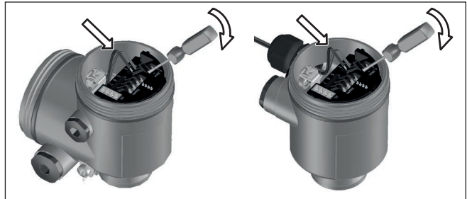
Abb. 20: Anschlusschritte 6 und 7
