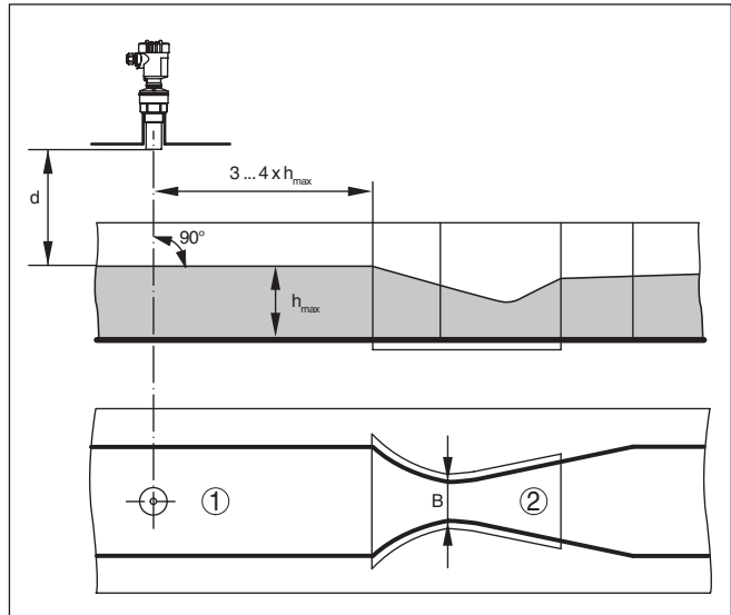
Abb. 19: Durchflussmessung mit Khafagi-Venturirinne: d = Blockdistanz des Sensors; h_{max} = max. Befüllung der Rinne; B = größte Einschnürung der Rinne
