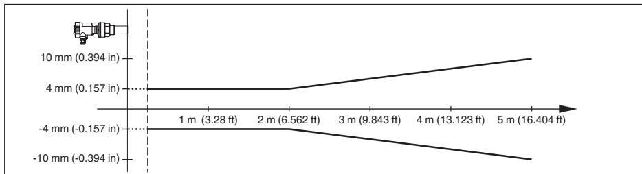
Abb. 36: Messabweichung VEGASON 61
