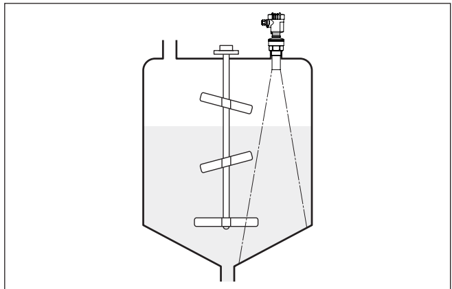
Abb. 15: Rührwerke
