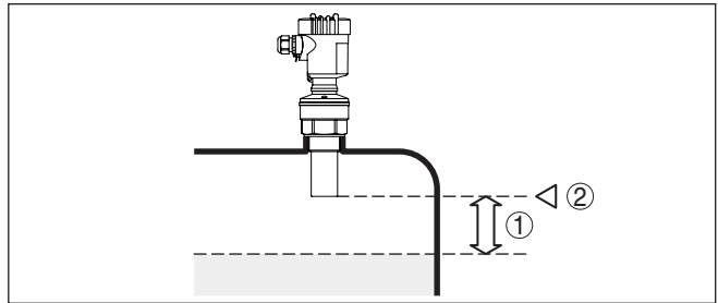
Abb. 6: Blockdistanz zur max. Füllhöhe
