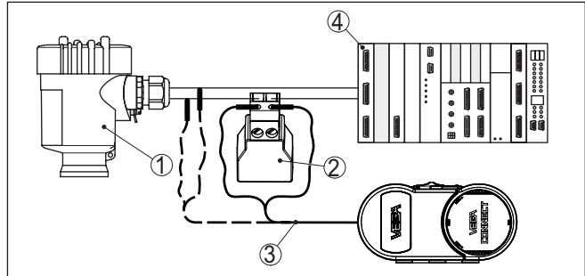
Abb. 34: Anschluss des PCs via HART an die Signalleitung
