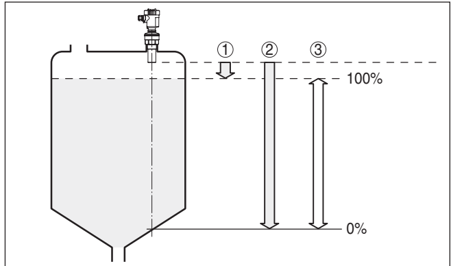
Abb. 7: Messbereich (Arbeitsbereich) und maximale Messdistanz
