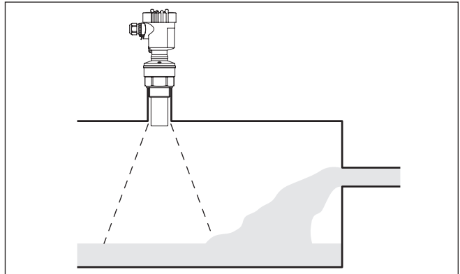
Abb. 16: Einströmende Flüssigkeit
