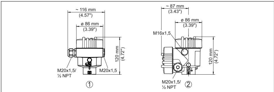
Abb. 38: Gehäuseausführungen in Schutzart IP68 (0,2 bar), (mit eingebautem Anzeige- und Bedienmodul vergrößert sich die Gehäusehöhe um 18 mm/0.71 in)
