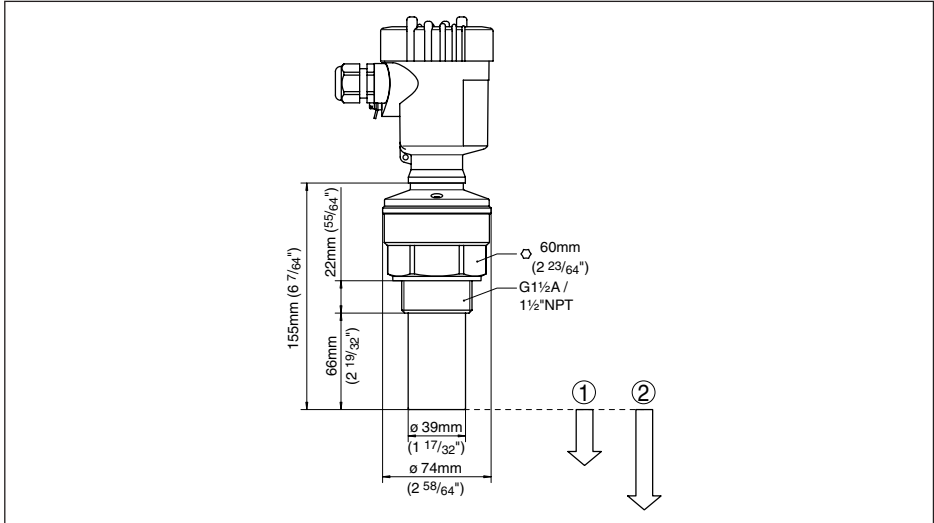
Abb. 42: VEGASON 61
