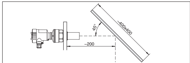
Abb. 13: Umlenkspiegel
