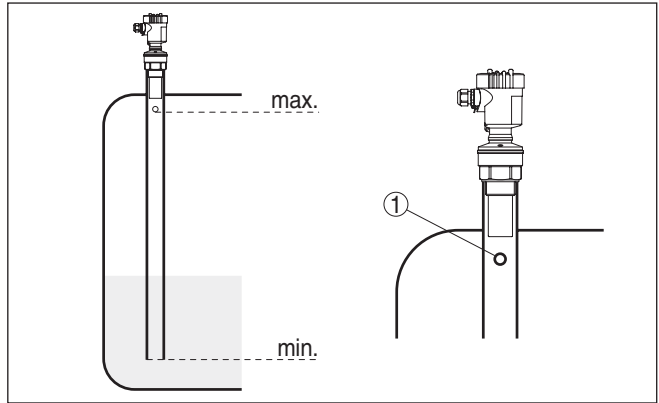
Abb. 17: Standrohr im Tank
