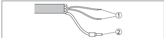
Abb. 28: Aderbelegung Anschlusskabel
