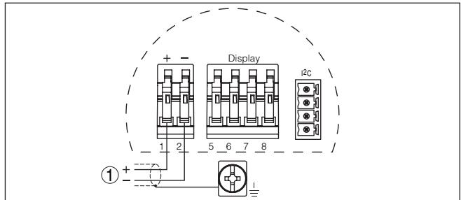
Abb. 23: Anschlussplan - Einkammergehäuse
