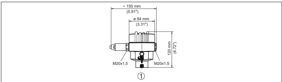
Abb. 41: Gehäuseausführungen in Schutzart IP66/IP68 (1 bar), (mit eingebautem Anzeige- und Bedienmodul vergrößert sich die Gehäusehöhe um 18 mm/0.71 in)
