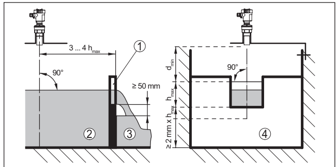
Abb. 18: Durchflussmessung mit Rechtecküberfall: d_{min} = Blockdistanz des Sensors (siehe Kapitel "Technische Daten"); h_{max} = max. Befüllung des Rechtecküberfalls
