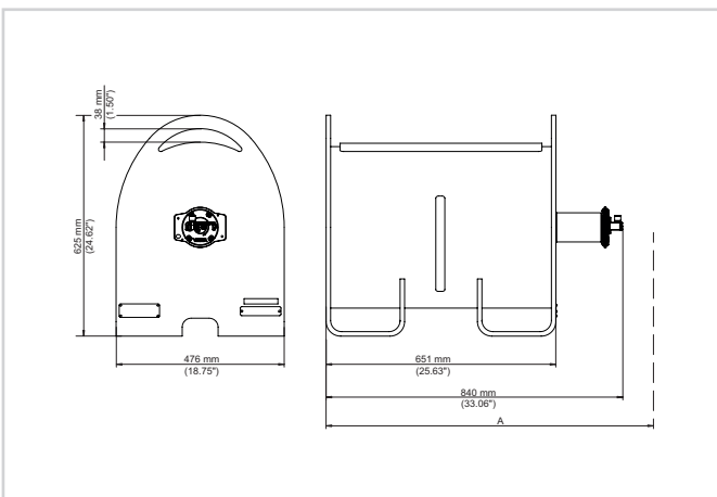
Dimensioni VEGASOURCE 86
