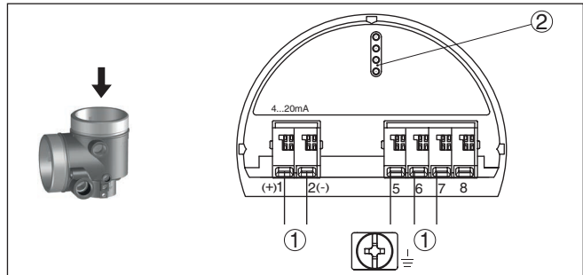
Fig. 6: Elektronicarimte - tweekamerbehuizing
