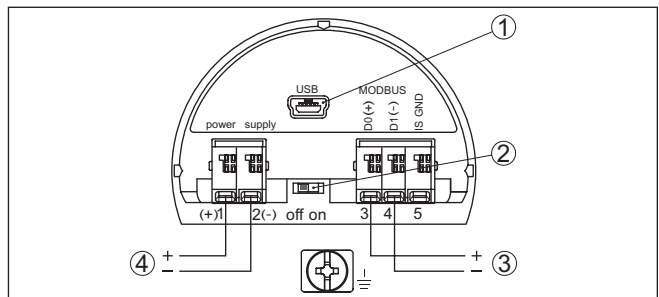
Figura 7: Vano di connessione
