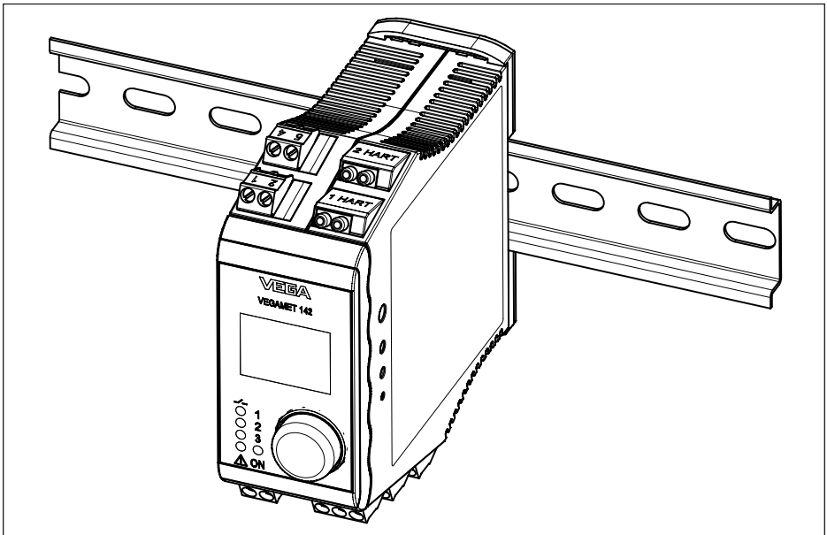
Сур. 1: VEGAMET 141, 142 на несущей рейке
