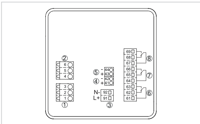
Aansluitschema VEGAMET 342
