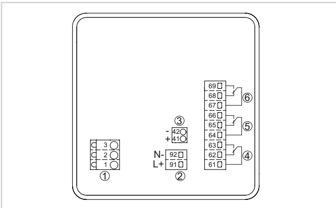
Aansluitschema VEGAMET 341
