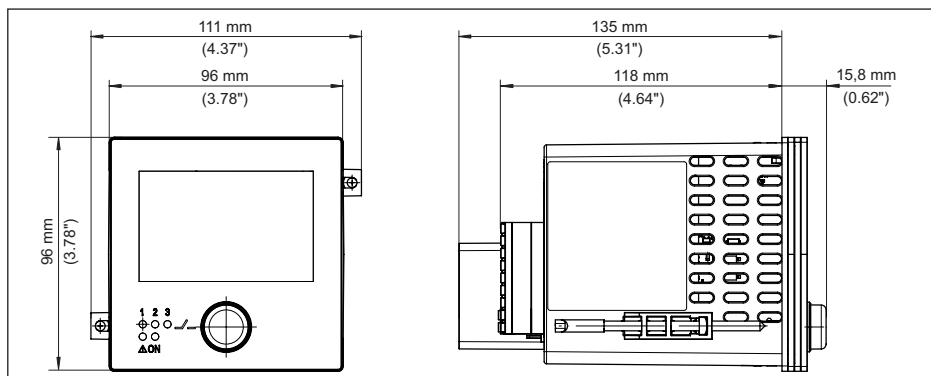
Fig. 23: Dimensões VEGAMET 342
