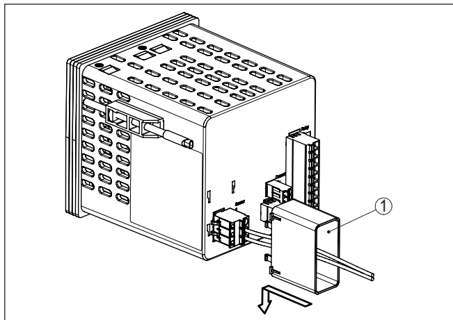
Fig. 7: Encaixar da câmara separadora Ex
