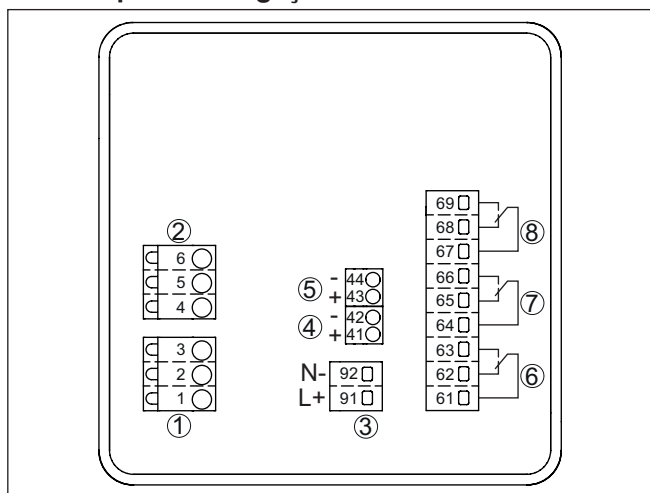
Fig. 4: Esquema de ligações VEGAMET 342
