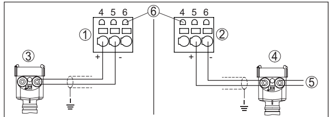
Fig. 6: Conexão entrada 2 para sensor de dois/quatro condutor (ativo/passivo)
