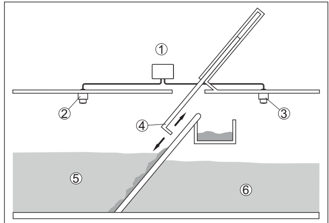
Fig. 20: Ejemplo de un control de vertedero
