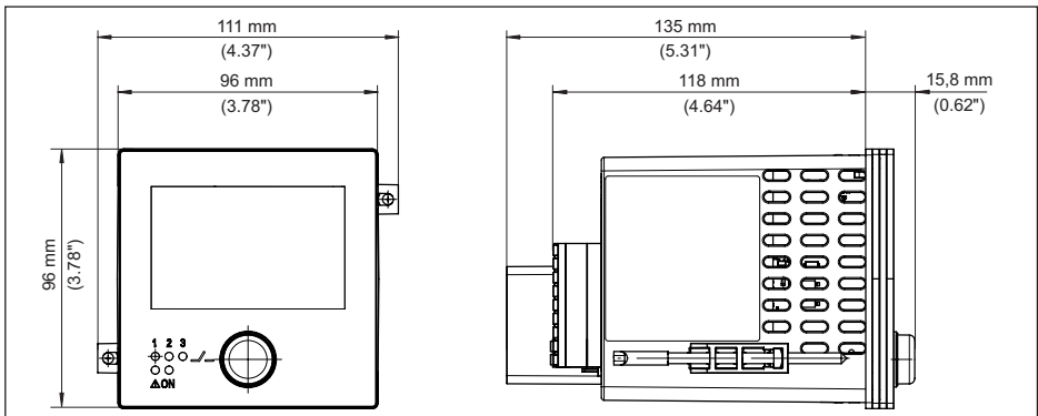
Fig. 23: Medidas VEGAMET 342
