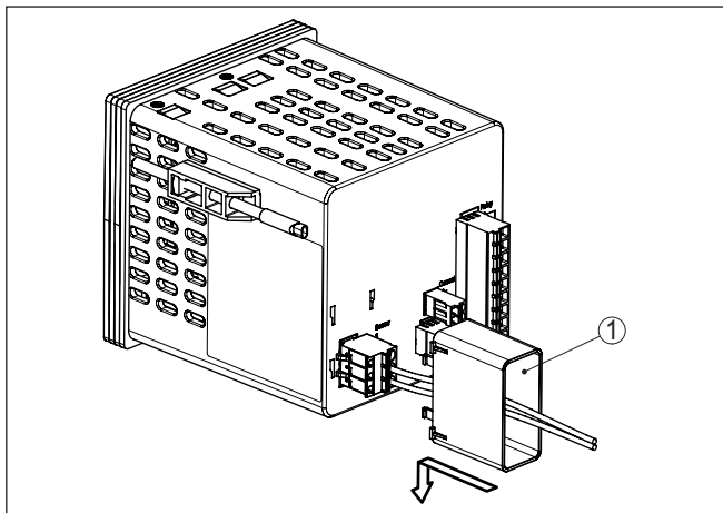
Fig. 7: Montaje de la cámara de separación Ex
