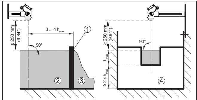
Fig. 21: Medición de caudal con canal rectangular: h_{max} = llenado máx. del canal rectangular
