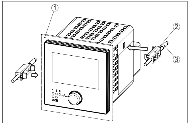
Fig. 3: Montaje en panel de control
