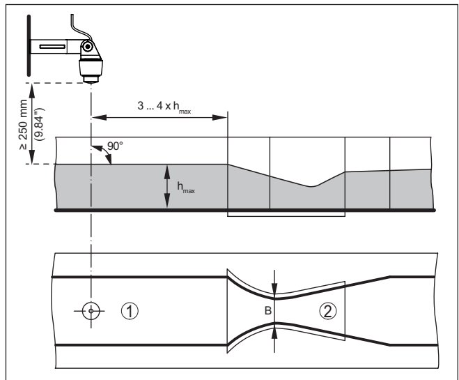
Fig. 22: Medición de caudal con canal venturi Khafagi: h_{max} = llenado máx. del canal; B = mayor estrechamiento del canal
