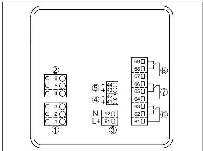
Fig. 4: Esquema de conexión VEGAMET 342
