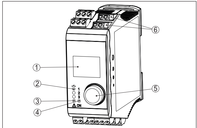
Fig. 6: Éléments de réglage et d'affichage
