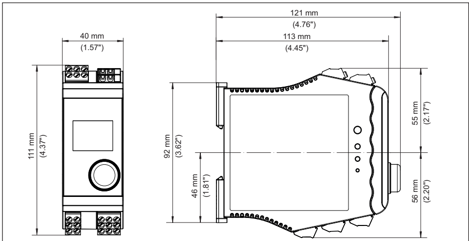
Fig. 21: Encombrement VEGAMET 142
