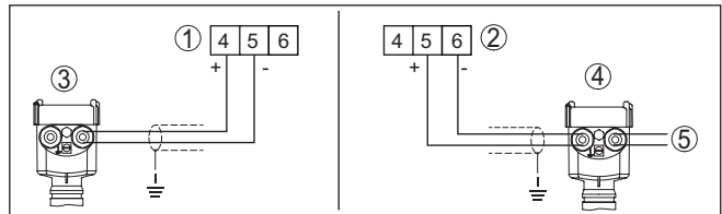
Fig. 5: Raccord entrée du capteur 2 pour capteur à deux fils/à quatre fils (actif/passif)
