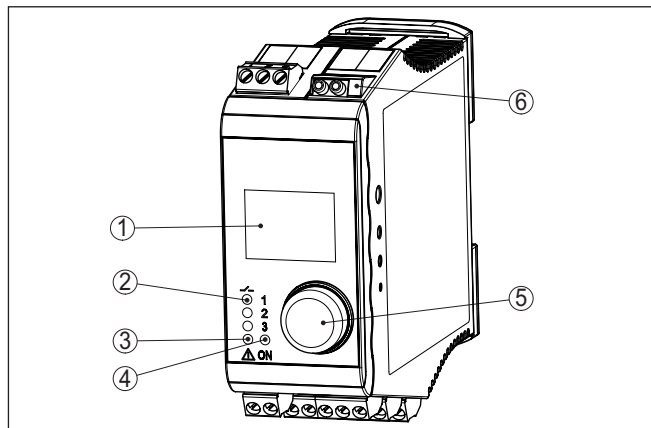
Rys. 5: Elementy obsługowe i wskaźniki
