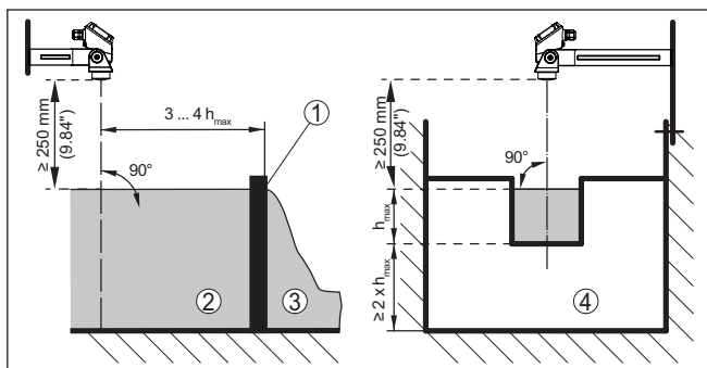
Rys. 17: Pomiar natężenia przepływu z przelewem prostokątnym: h_{\text{max}} = \text{max} . napelnienie przelewu prostokątnego
