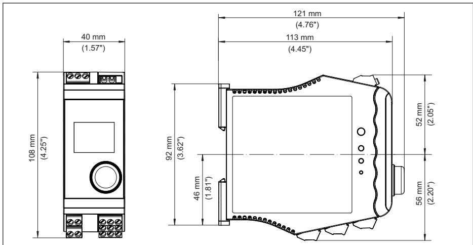
Rys. 19: Wymiary VEGAMET 141
