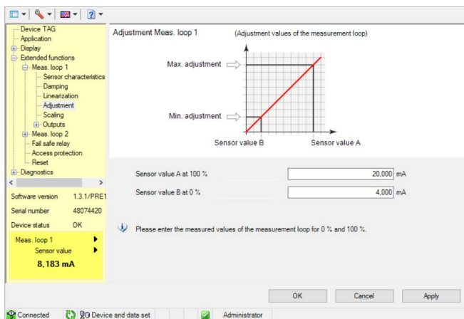
Rys. 9: Przykładowy widok DTM - kompensacja
