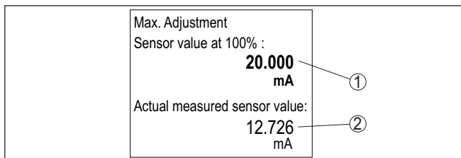
Rys. 7: Przykład widoku opcji menu: kompensacja max.
