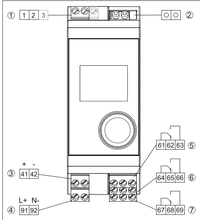
Rys. 3: Schemat przyłączy VEGAMET 141
