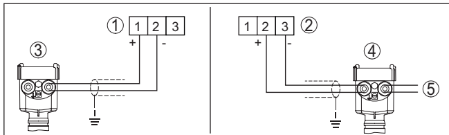
Rys. 4: Przyłącze wejścia dla sondy w systemie dwuprzewodowym/czterprzewodowym (aktywna/pasywna)
