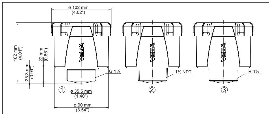
Figura 29: Dimensioni VEGAPULS Air 41
