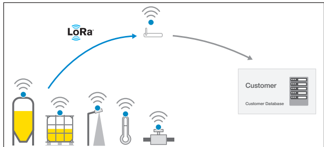
Figura 18: Trasmissione wireless dei valori di misura
