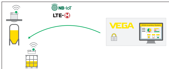
Figura 25: Accesso remoto al sensore dal VEGA Inventory System tramite NB-IoT o LTE-M
