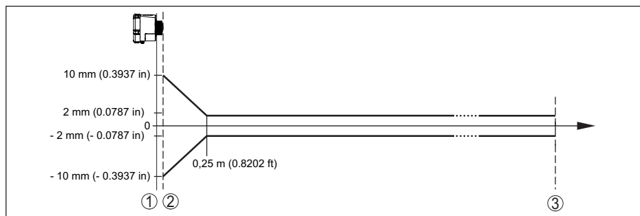
Figura 28: Scostamento di misura sotto condizioni di riferimento
