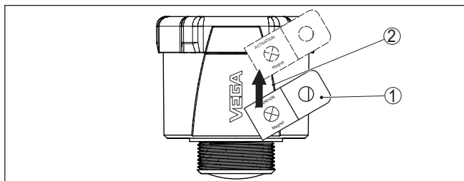
Figura 14: Attivazione del sensore tramite magnete
