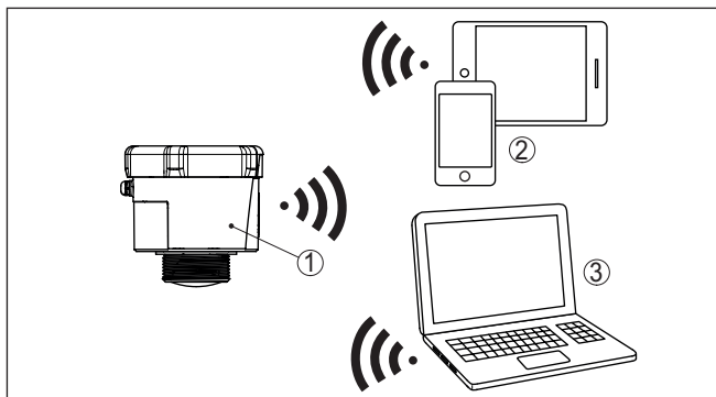
Figura 3: Collegamento wireless a strumenti di calibrazione standard tramite Bluetooth
