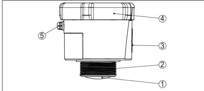
Figura 1: Componenti del sensore VEGAPULS Air 41 - esempio: esecuzione con filettatura G1½
