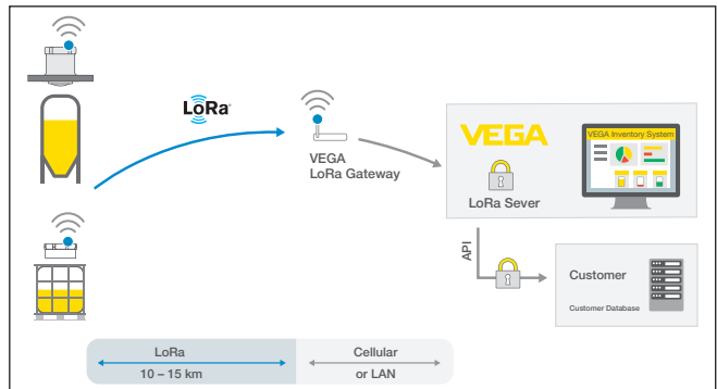
Figura 16: Trasmissione wireless dei valori di misura tramite LoRa-WAN, server LoRa al VEGA Inventory System
