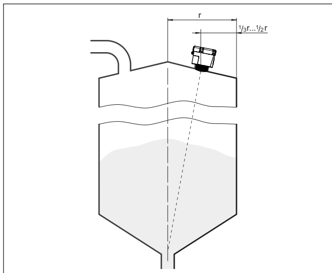
Figura 11: Posizione di montaggio e orientamento
