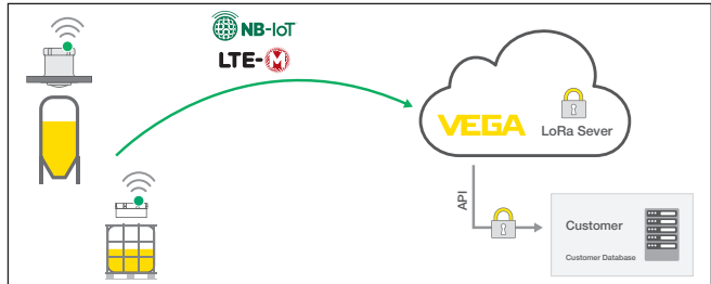
Figura 17: Trasmissione wireless dei valori di misura al cloud di VEGA tramite NB-IoT e LTE-M
