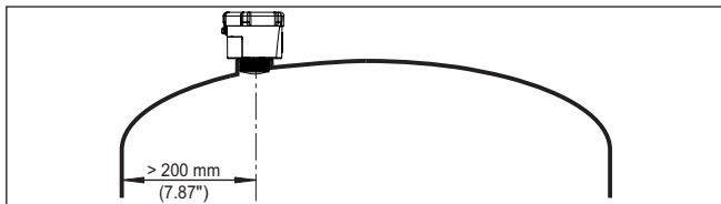
Figura 5: Montaggio del sensore radar su un cielo del serbatoio bombato
