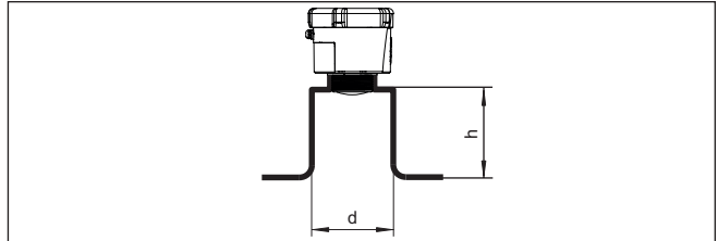
Figura 9: Montaggio su tronchetto in caso di dimensioni diverse del tronchetto
