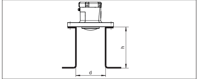
Res. 9: Boru soketleri ebatları standarttan farklı olduğunda
