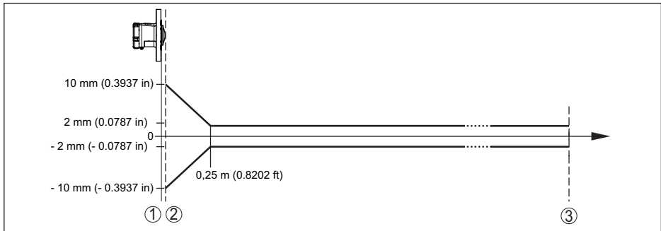
Res. 28: Referans koşullarına tabi ölçüm sapması
