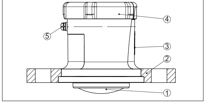
Res. 1: VEGAPULS Air 42 sensörünün bileşenleri (DN 80 sıkıştırma flanşlı model)
