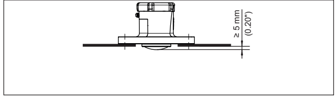
Res. 8: VEGAPULS Air 42 cihazının tavsiye edilmeye değer boru soketi montajı
