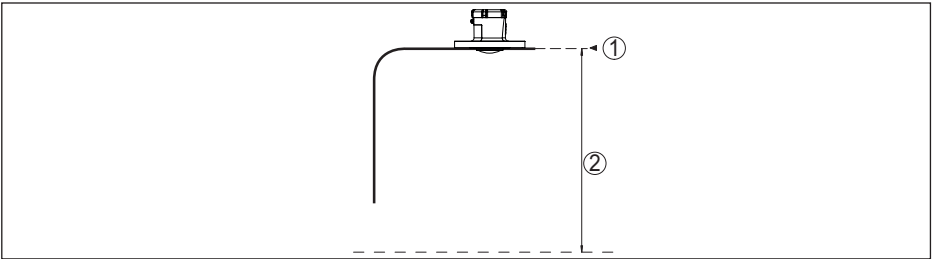
Res. 27: Giriş büyüklüğü ile ilgili veriler
