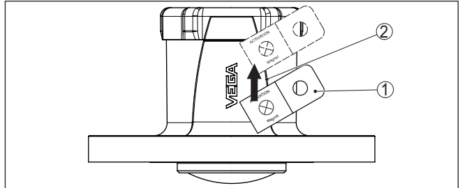
Res. 14: Sensörün mıknatıs ile etkinleştirilmesi
