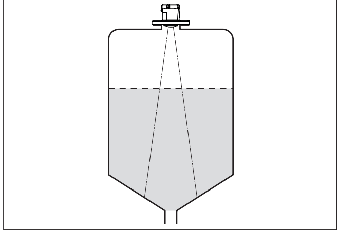
Res. 6: Radar sensörünün konik tabanlı haznelere montajı
