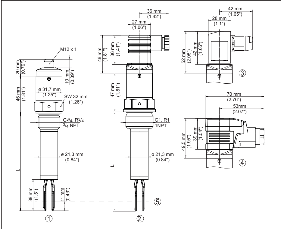
Res. 18: VEGASWING 53, Standart model, Dişli bağlantılar
