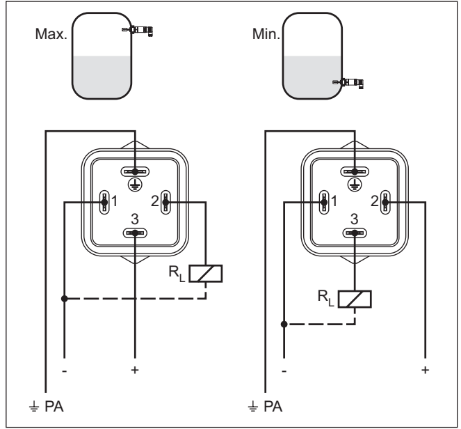
Res. 13: Bağlantı planı, ventilli fiş ISO 4400'de transistör çıkışı
