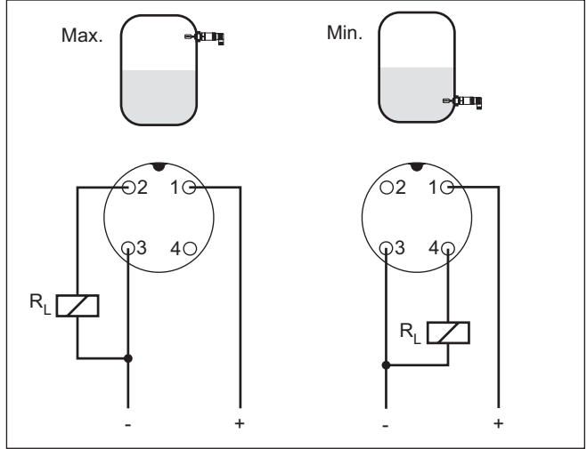
Res. 14: Bağlantı planı (gövde), M12 x 1 fiş bağlantısında transistör çıkışı
