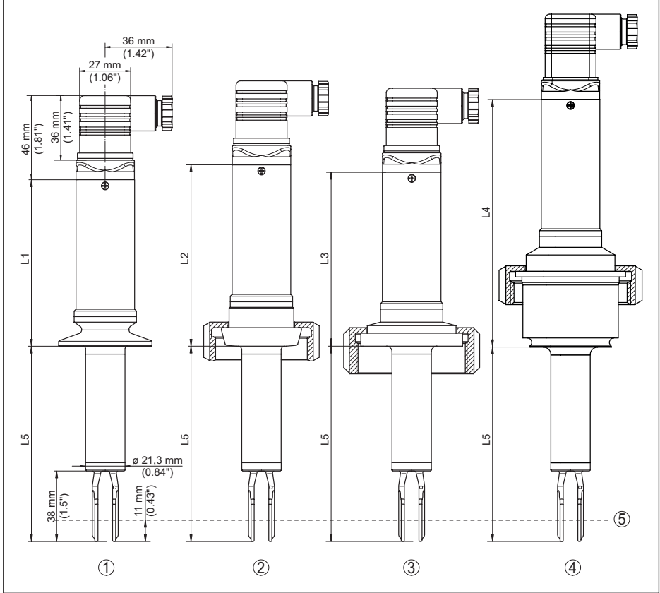
Res. 20: VEGASWING 53, Gıda malzemesi modelleri, Hijyenik bağlantılar
