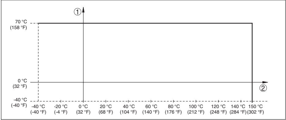
Res. 17: Çevre sıcaklığının proses sıcaklığına bağımlılığı
