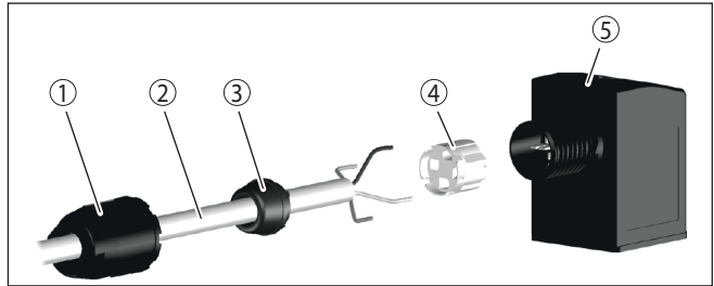
Rys. 7: Połączenie wtyczki do zaworów ISO 4400 z połączeniem zaciskowym IDC
