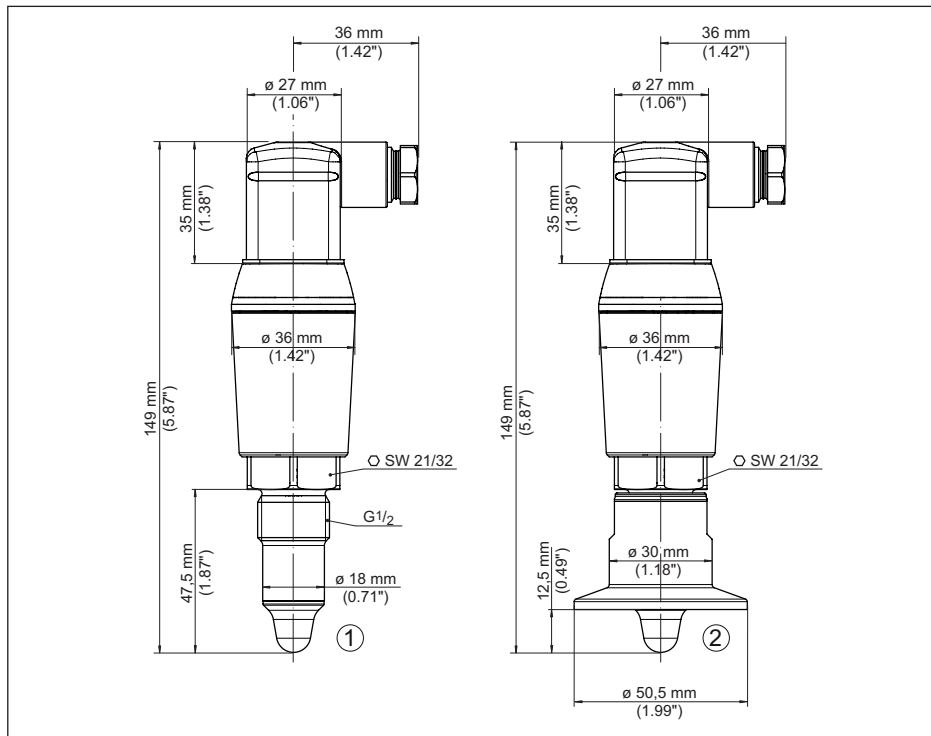
Rys. 19: VEGAPOINT 31, wersja sterylna - gwint z wtyczką ISO 4400
