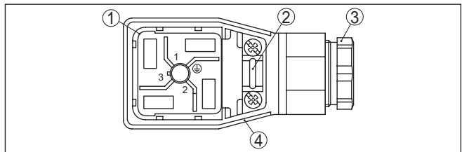
Rys. 8: Odłączenie wkładki wtyczki
