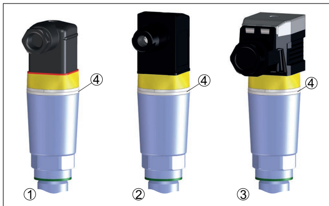
Rys. 5: Wersje wykonania wtyczek
