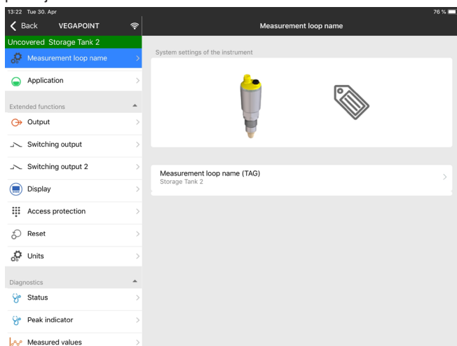
Rys. 14: Przykładowy widok aplikacji - rozruch
