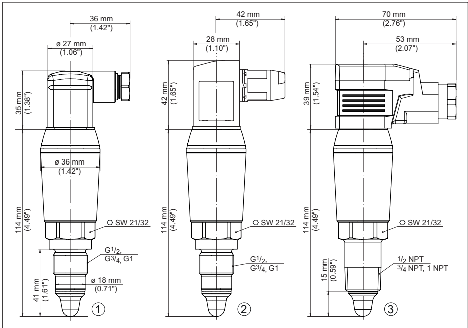
Rys. 18: VEGAPOINT 31, wersja standardowa - gwint z wtyczką do zaworów według ISO 4400
