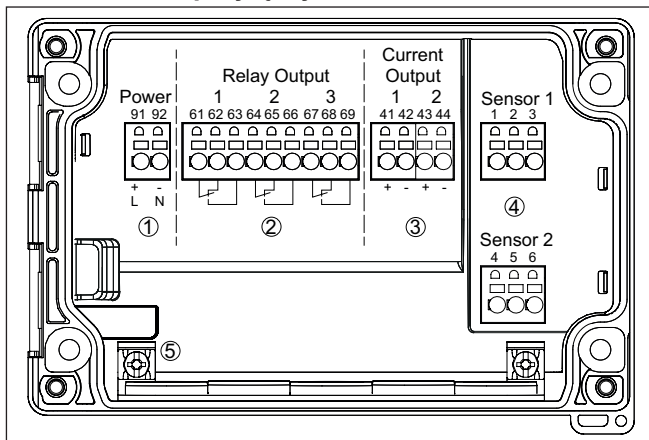
Rys. 6: Schemat przyłączy VEGAMET 842
