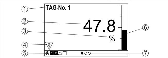
Rys. 10: Przykład wyświetlania zmierzonej wartości (wartość pomiarowa z wykresem słupkowym)
