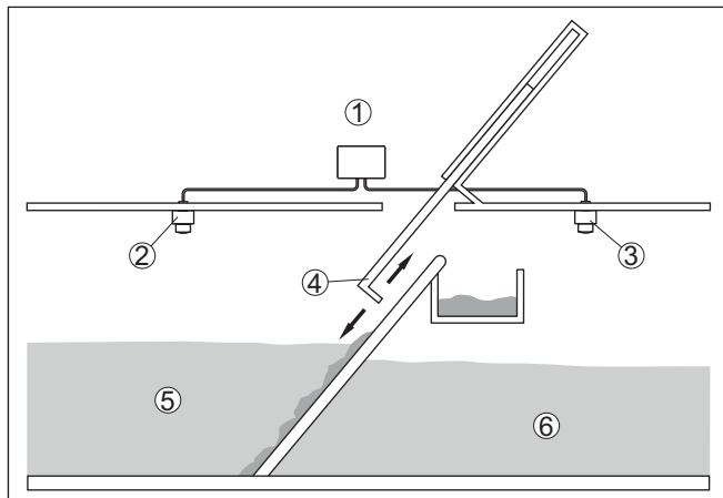
Rys. 21: Przykład sterownika zabieraka
