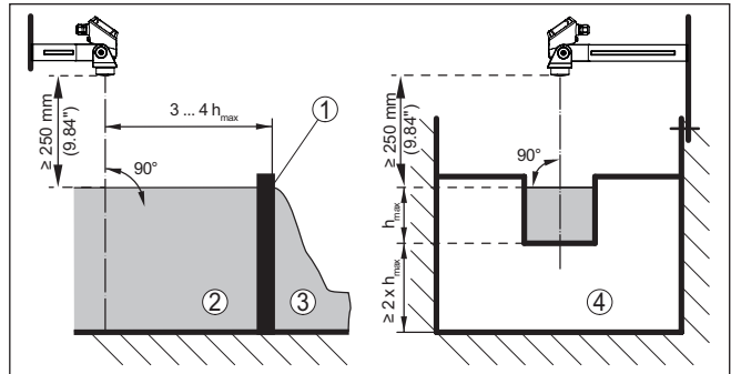
Rys. 22: Pomiar natężenia przepływu z przelewem prostokątnym: h_{max} = max. napelnienie przelewu prostokątnego
