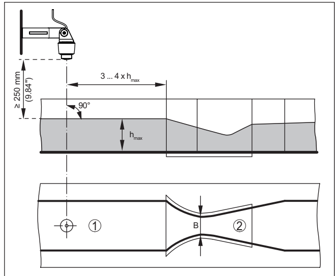
Rys. 23: Pomiar natężenia przepływu z użyciem zwężki Venturiego: h_{max} = max. napelnienie kanału; B = największe zwężenie kanału
