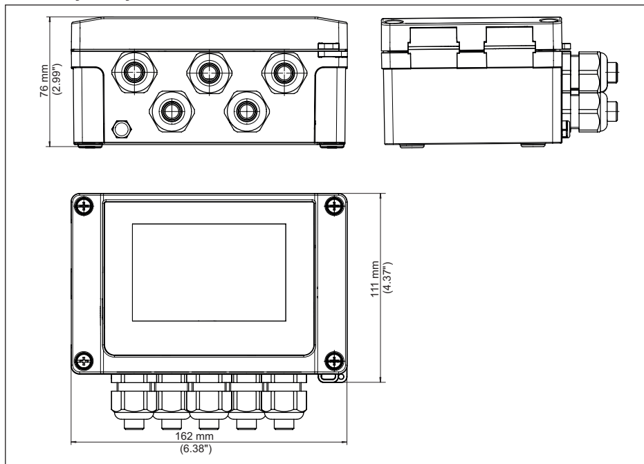
Rys. 24: Wymiary VEGAMET 842
