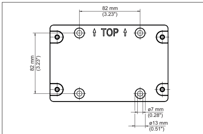
Rys. 3: Płyta do montażu ściennego VEGAMET 842
