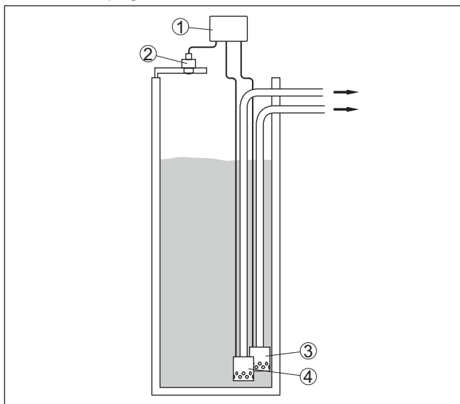
Rys. 15: Przykładowa stacja pomp: sterowanie pracą pomp w studzience wlotowej
