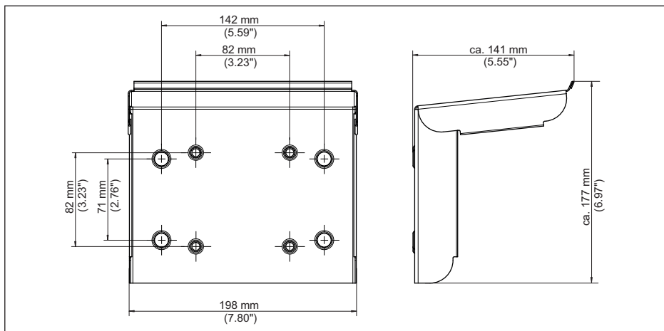
Rys. 26: Wymiary osłony przed nastonecznieniem
