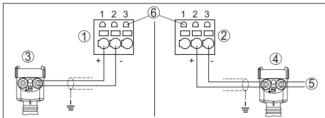
Rys. 7: Przyłącze wejścia 1 dla sondy w systemie dwuprzewodowym/czterprzewodowym (aktywna/pasywna)
