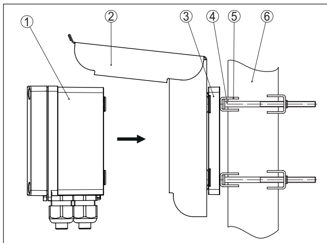
Rys. 5: Montaż osłony przed nasłonecznieniem przy montażu rurze
