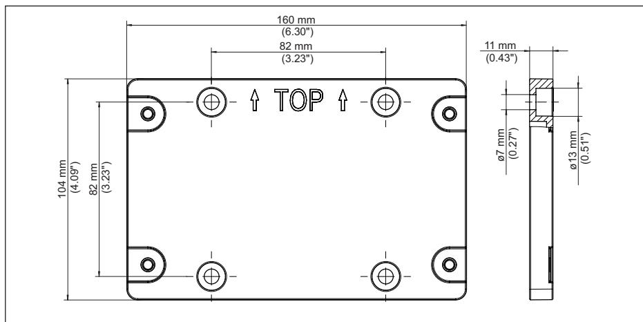
Rys. 25: Wymiary płyty montażowej
