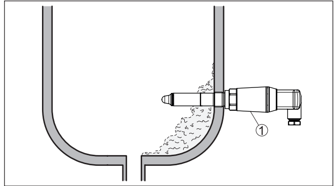
Fig. 5: Montagem lateral - Sedimentações 1 VEGAPOINT 23, montado lateralmente
