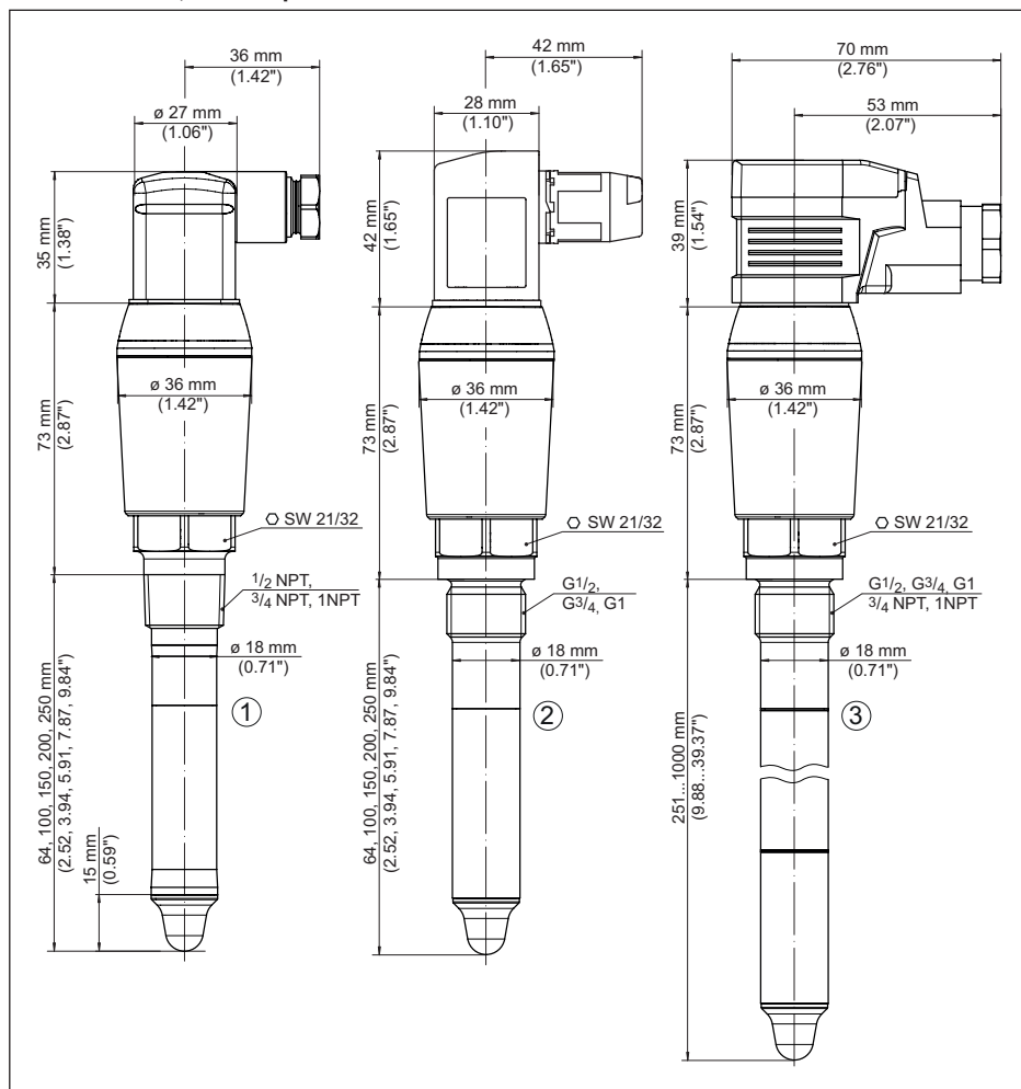
Fig. 20: VEGAPOINT 23, modelo padrão - Rosca, com conector de válvula conforme ISO 4400
