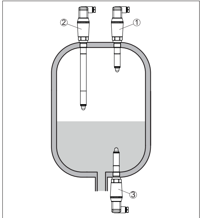
Fig. 4: Exemplos de montagem
