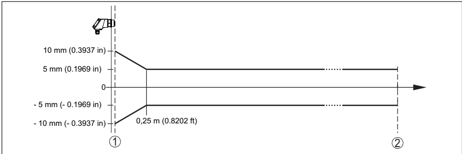
Fig. 27: Écart de mesure sous conditions de référence 9)
