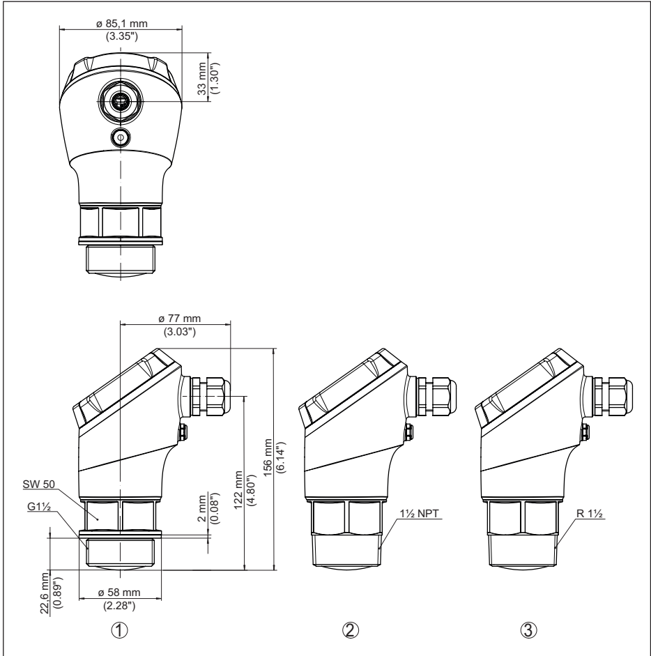
Fig. 28: Encombrement VEGAPULS 11
