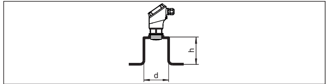
Fig. 10: Montage sur rehausse
