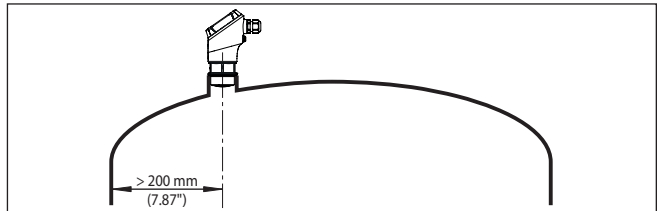
Fig. 5: Montage du capteur radar dans une cuve à toit bombé
