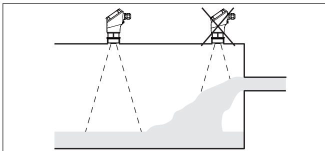
Fig. 8: Montage du capteur radar en présence d'un flux de produit
