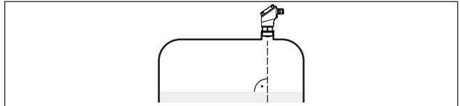
Fig. 12: Orientation du capteur dans les liquides
