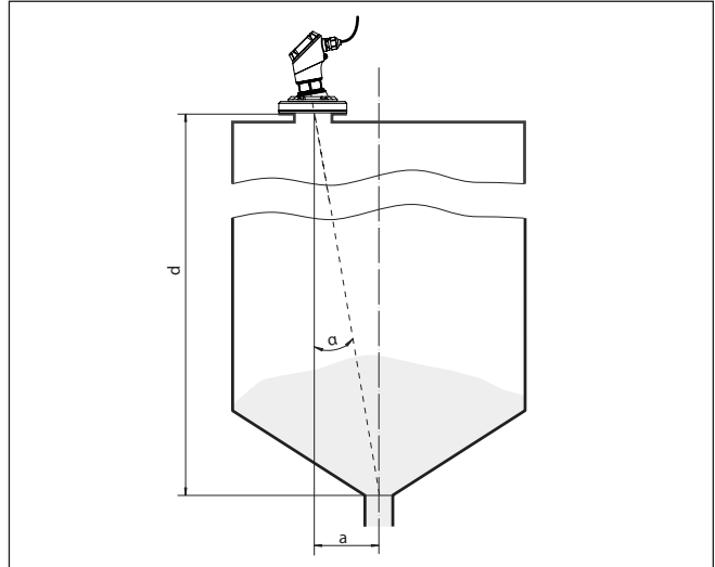
Fig. 14: Proposition pour un montage après orientation VEGAPULS 11
