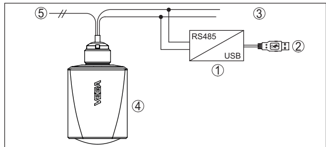
Fig. 23: Aansluiting van de PC op de signaalkabel
