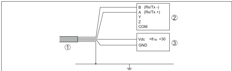
Fig. 28: Aansluiting van de VEGAPULS C 23 op RTU Fisher ROC 809
