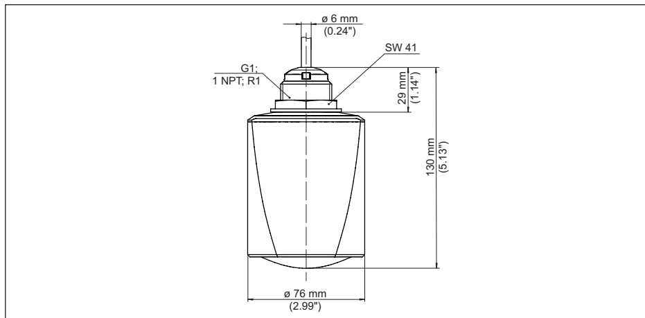
Fig. 29: Afmetingen VEGAPULS C 23
