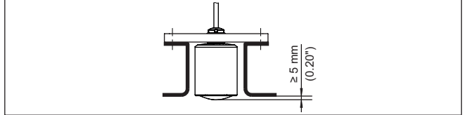
Figura 11: Montaggio su tronchetto consigliato del VEGAPULS C 23
