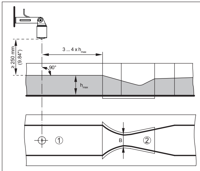
Figura 17: Misura di portata con canale Khafagi-Venturi: h_{max} = max. riempimento del canale; B = massima strozzatura del canale
