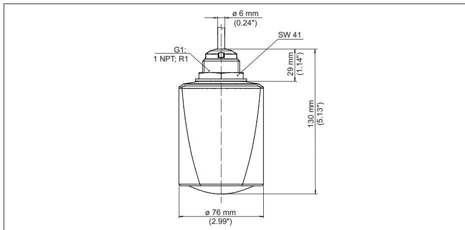
Figura 29: Dimensioni VEGAPULS C 23
