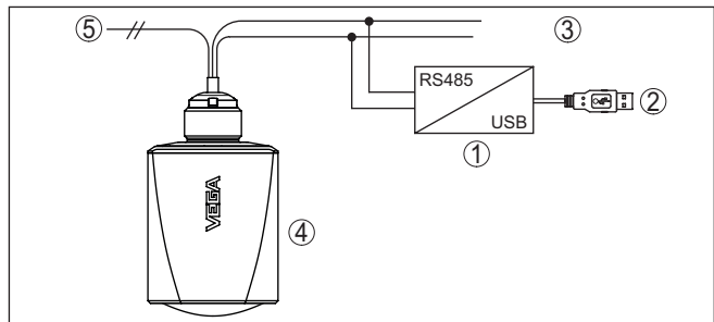
Figura 23: Collegamento del PC alla linea del segnale
