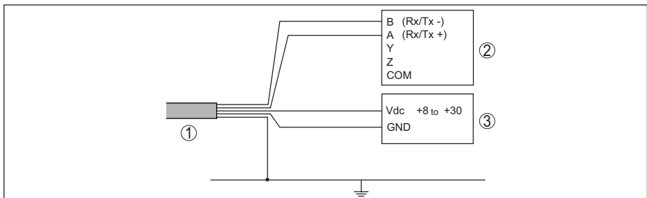
Figura 28: Collegamento del VEGAPULS C 23 a RTU Fisher ROC 809
