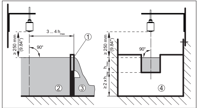
Figura 16: Misura di portata con stramazzone rettangolare: h_{max.} = max. riempimento dello stramazzone rettangolare
