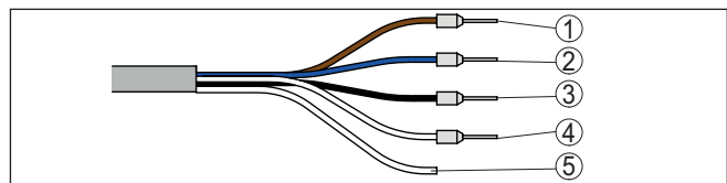
Figura 18: Assegnazione dei conduttori del cavo di connessione collegato fisso
