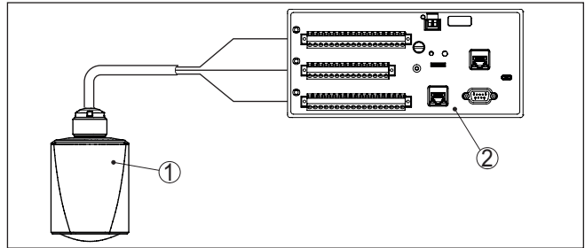
Fig. 4: Conexión del VEGAPULS C 23 SDI-12 al registrador de datos
