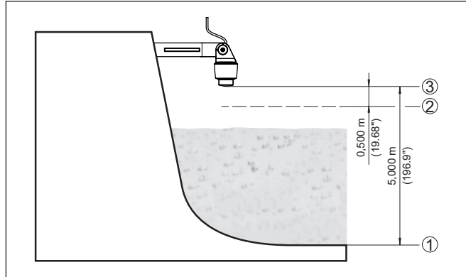
Fig. 24: Ejemplo de parametrización ajuste mín/máx
