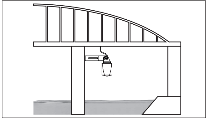
Fig. 14: Medición de nivel de río, montaje de sensor en pilar de puente
