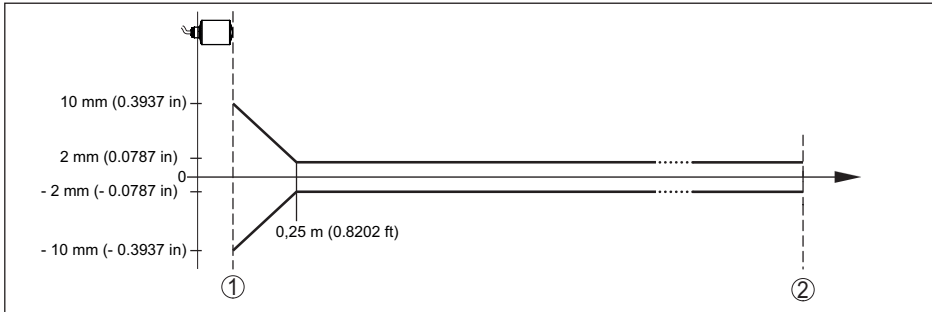
Fig. 27: Error de medición bajo condiciones de referencia 9)
