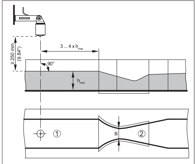
Fig. 18: Medición de caudal con canal venturi Khafagi; h_{max} = llenado máx. del canal; B = mayor estrechamiento del canal
