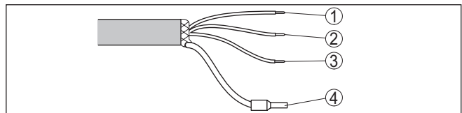
Fig. 19: Dotación de conductores, cable de conexión de conexión fija
