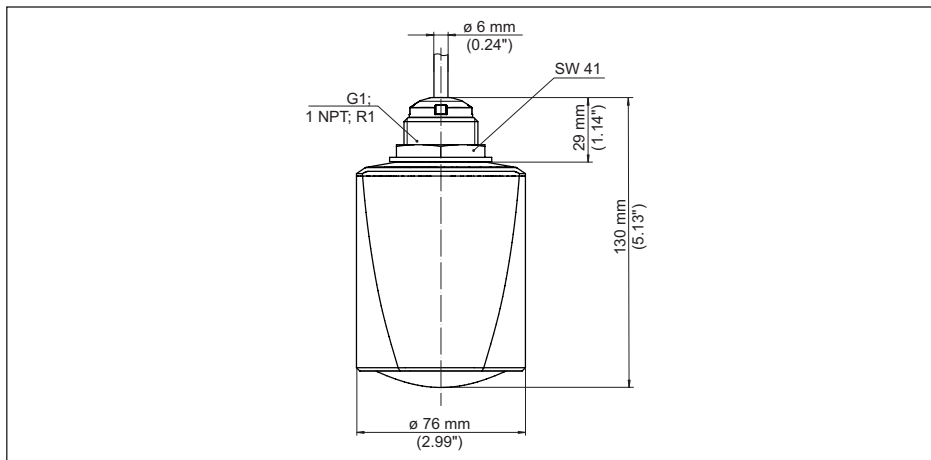
Fig. 28: Medidas VEGAPULS C 23
