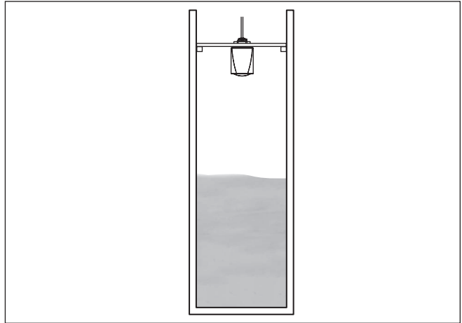
Fig. 16: Medición de nivel de pozo profundo, montaje de sensor en tapa
