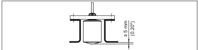
Fig. 9: Montaje recomendado en tubuladura del VEGAPULS C 23
