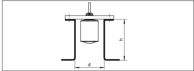
Fig. 10: Montaje de tubuladuras con medidas divergentes
