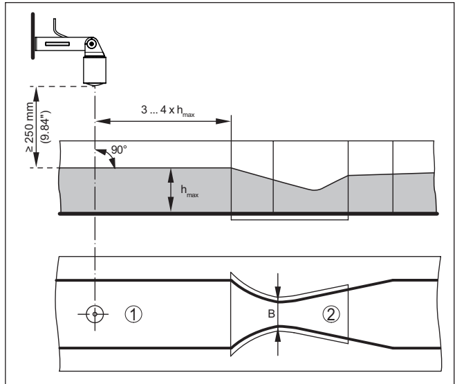
Fig. 18: Flowmeting met Khafagi-venturigoot: h_{max} = max. peil in de goot; B = maximale insnoering van de goot
