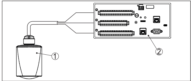
Fig. 4: Aansluiting van de VEGAPULS C 23 SDI-12 op de datalogger
