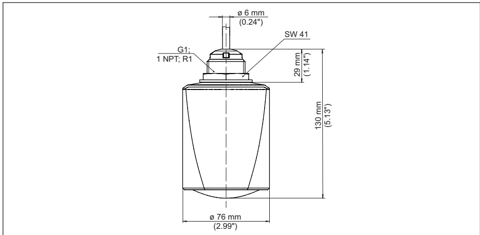
Fig. 28: Afmetingen VEGAPULS C 23
