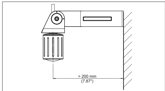
Fig. 5: Montage via een montagehoekstuk
