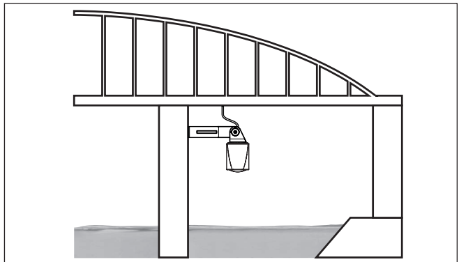
Fig. 14: Peilmeting rivier, sensormontage op brugpijler
