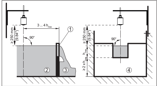
Fig. 17: Flowmeting met rechthoekig overstortschot: h_{max} = max. vulling van het rechthoekig overstortschot
