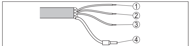
Fig. 19: Aderbezetting vast aangesloten aansluitkabel
