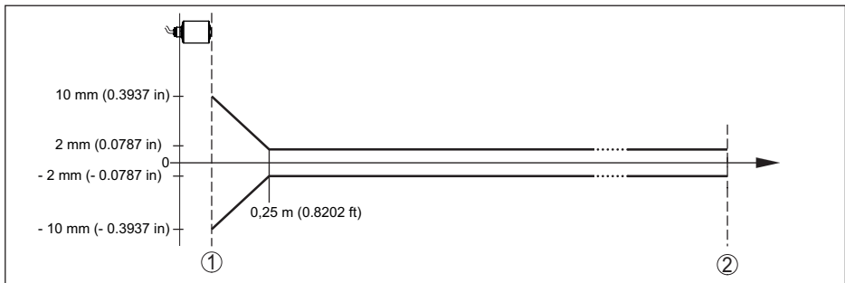
Fig. 27: Meetnauwkeurigheid onder referentiecondities 9)
