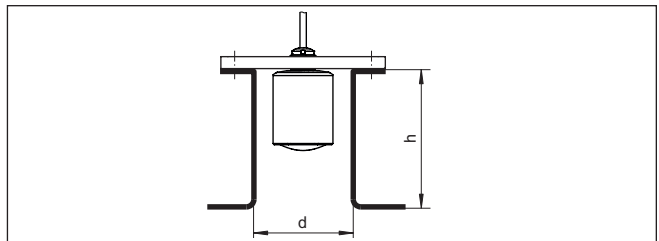
Fig. 10: Sokmontage bij afwijkende afmetingen
