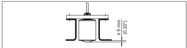
Fig. 9: Aanbevolen montage sok van de VEGAPULS C 23
