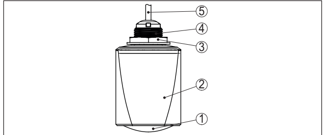
Fig. 1: Componentes del VEGAPULS C 23
