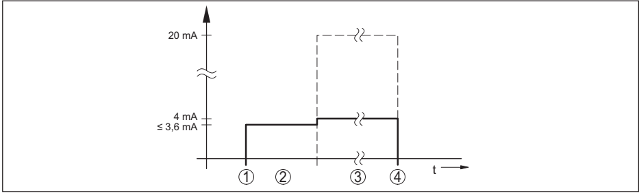
Fig. 29: Tiempo de aceleración y salida del valor de medición
