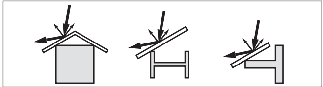
Fig. 13: Tapar los perfiles lisos con pantallas dispersoras
