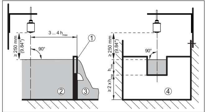
Fig. 18: Medición de caudal con canal rectangular: h_{max} = llenado máx. del canal rectangular
