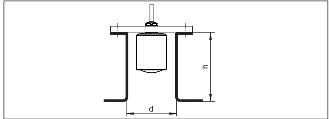
Fig. 12: Montaje de tubuladuras con medidas divergentes
