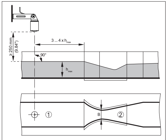
Fig. 19: Medición de caudal con canal venturi Khafagi: h_{max} = llenado máx. del canal; B = mayor estrechamiento del canal
