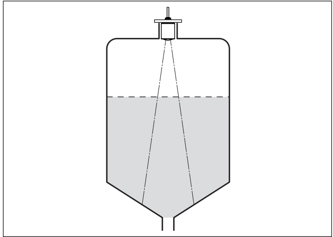
Fig. 8: Montaje del sensor de radar en depósito con fondo cónico
