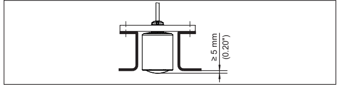
Fig. 11: Montaje recomendado en tubuladura del VEGAPULS C 23
