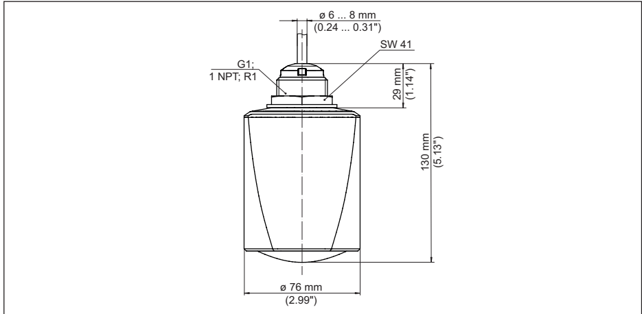
Fig. 32: Medidas VEGAPULS C 23
