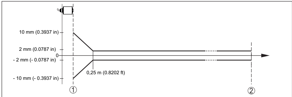
Fig. 31: Error de medición bajo condiciones de referencia 9)
