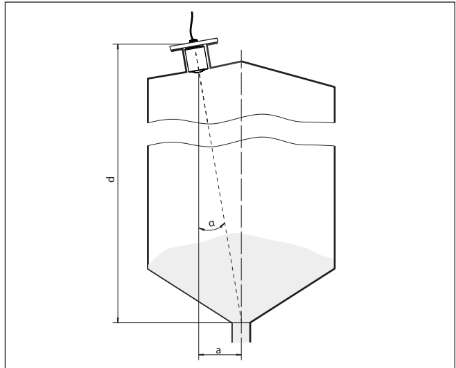
Fig. 16: Propuesta de montaje después de la orientación VEGAPULS C 23
