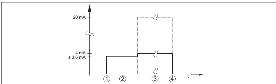
Fig. 29: Opstarttijd en uitsturen meetwaarde
