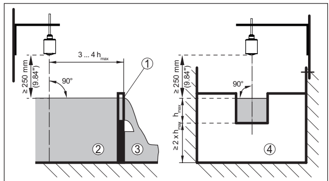
Fig. 18: Flowmeting met rechthoekig overstortschot: h_{\text{max}} = max. vulling van het rechthoekig overstortschot
