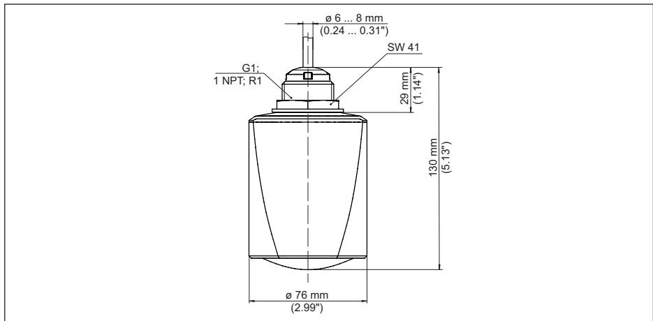
Fig. 32: Afmetingen VEGAPULS C 23
