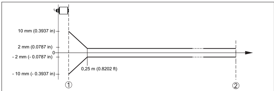
Abb. 31: Messabweichung unter Referenzbedingungen 1)
