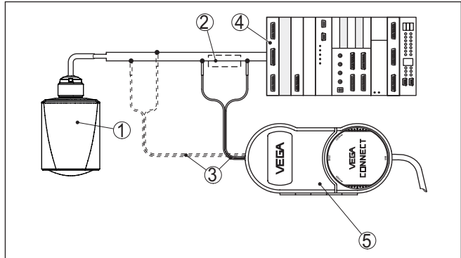
Abb. 25: Anschluss des PCs an die Signalleitung
