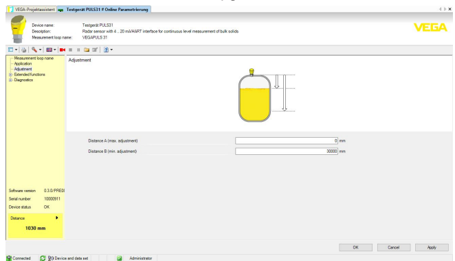
Fig. 25: Voorbeeld van een DTM-aanzicht - inbedrijfname sensorinregeling
