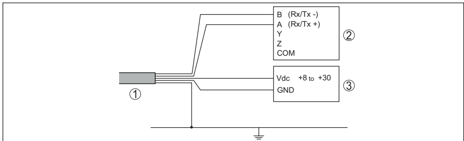
Fig. 31: Aansluiting van de VEGAPULS C 22 op RTU Fisher ROC 809
