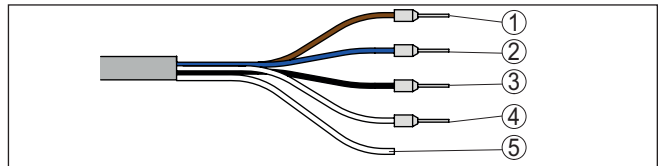
Fig. 21: Aderbezetting vast aangesloten aansluitkabel
