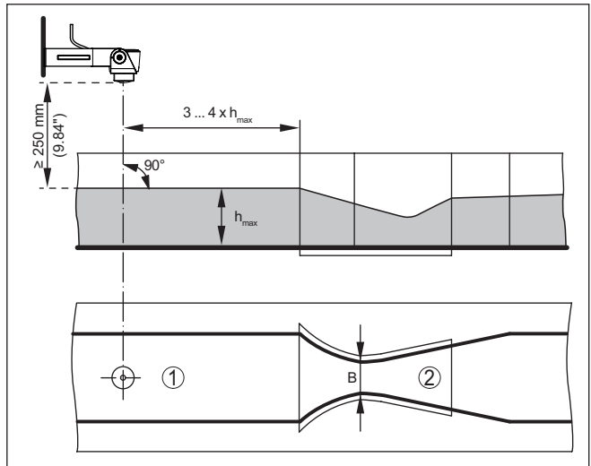
Fig. 20: Flowmeting met Khafagi-venturigoot: h_{max} = max. peil in de goot; B = maximale insnoering van de goot
