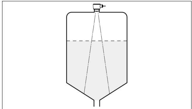
Fig. 9: Montage van de radarsensor op tanks met conische bodem
