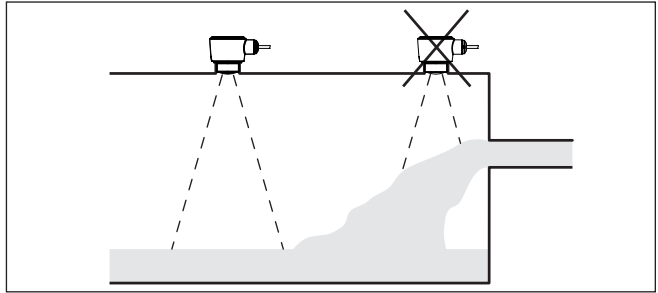
Fig. 11: Montage van de radarsensor bij instromend product
