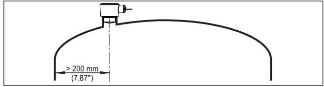
Fig. 8: Montage van de radarsensor op ronde tankdaken
