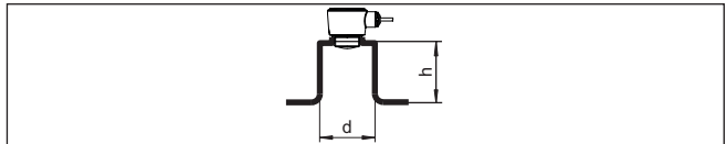
Fig. 13: Sokmontage bij afwijkende afmetingen
