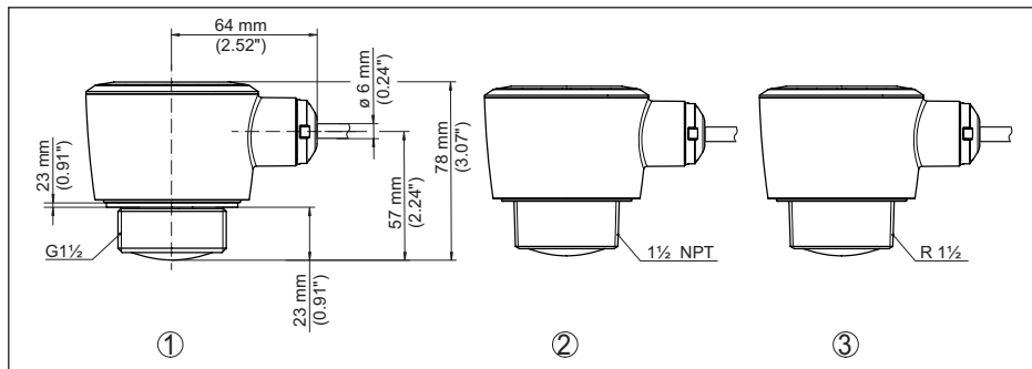
Fig. 32: Afmetingen VEGAPULS C 22
