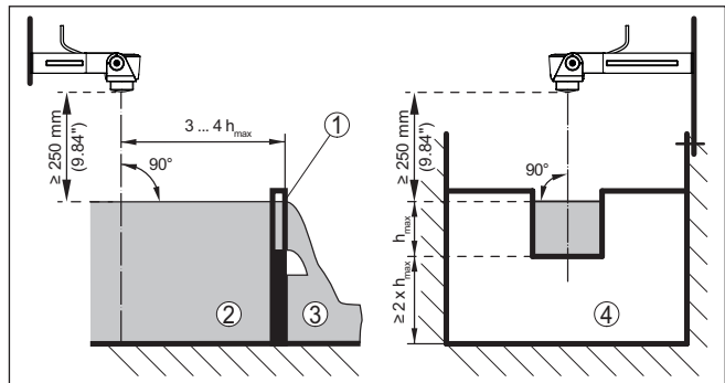
Rys. 18: Pomiar natężenia przepływu z przelewem prostokątnym: h_{\text{max}} = \text{max} . napelnienie przelewu prostokątnego
