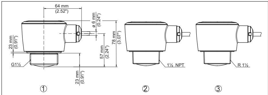
Rys. 29: Wymiary VEGAPULS C 22
