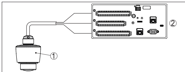
Rys. 4: Podłączenie VEGAPULS C 22 SDI-12 do rejestratora przemysłowego
