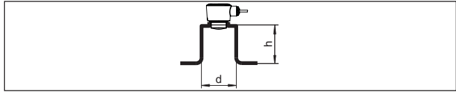
Rys. 11: Montaż króćca rurowego przy innych wymiarach króćca rurowego
