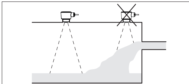
Rys. 9: Montaż sondy radarowej przy wpływającym medium
