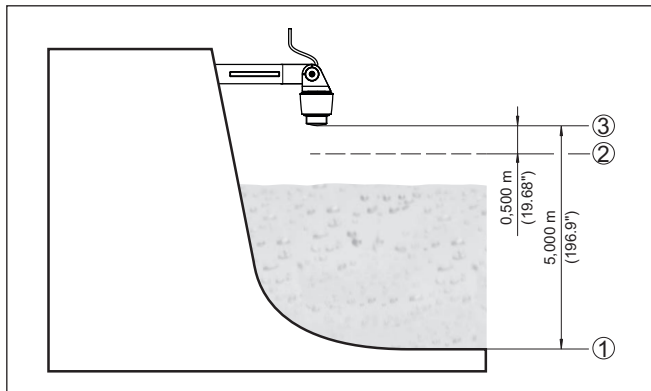
Rys. 25: Przykładowe parametry kompensacji min./max.
