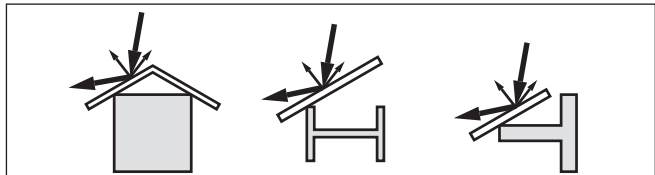
Rys. 12: Gładkie profile ostionić blachami rozpraszającymi
