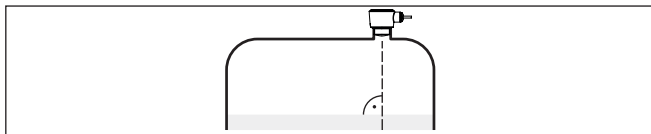
Rys. 13: Ukierunkowanie w przypadku ciecży
