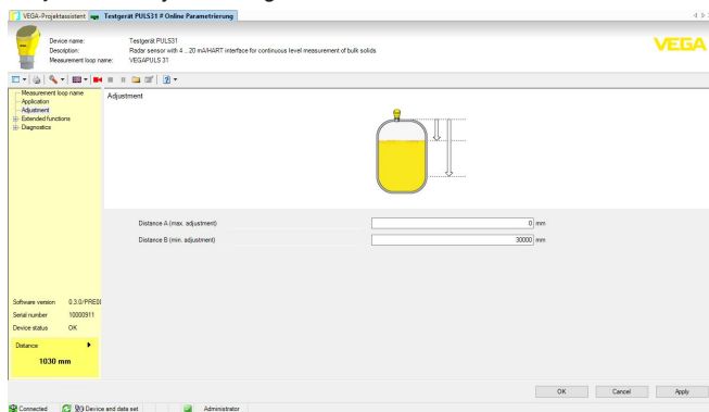
Rys. 24: Przykładowy obraz DTM rozruchu - dostrojenie sondy
