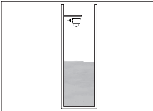
Rys. 17: Pomiar poziomu w studni głębinowej, montaż sondy na pokrywie
