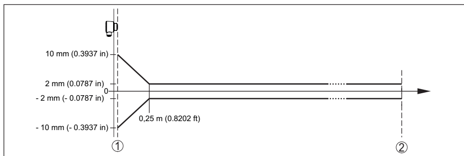
Rys. 28: Odchyłka pomiarowa w warunkach referencyjnych 10)
