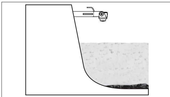
Rys. 16: Pomiar poziomu przy zaporze, montaż sondy na wysięgniku
