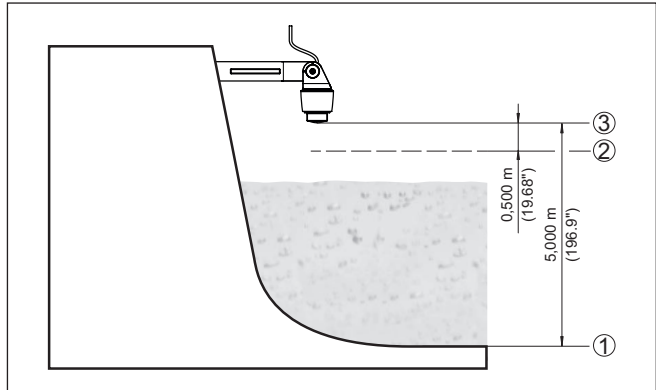
Fig. 25: Parametreevoorbeeld min./max.-inregeling
