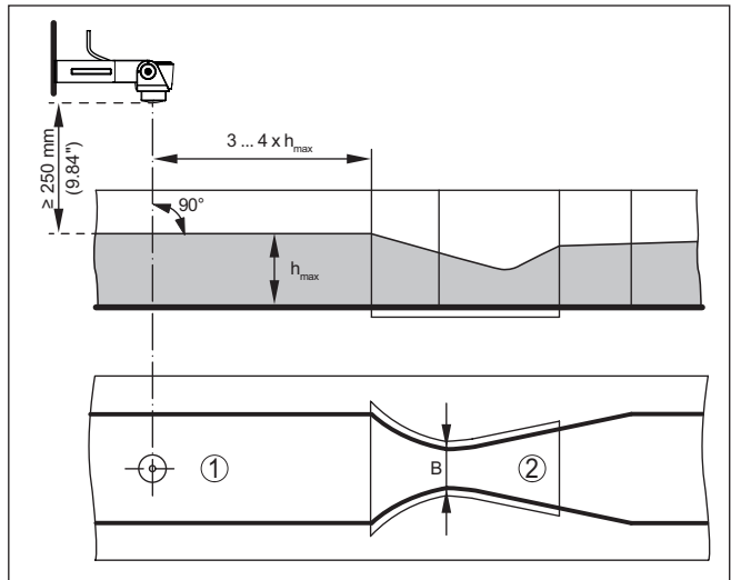
Fig. 19: Flowmeting met Khafagi-venturigoot: h_{max} = max. peil in de goot; B = maximale insnoering van de goot
