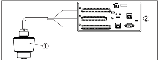
Fig. 4: Aansluiting van de VEGAPULS C 22 SDI-12 op de datalogger
