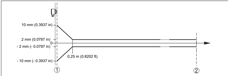
Fig. 28: Meetnauwkeurigheid onder referentiecondities 10)
