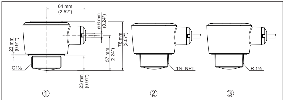
Fig. 29: Afmetingen VEGAPULS C 22
