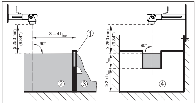
Fig. 18: Flowmeting met rechthoekig overstortschot: h_{\text{max}} = max. vulling van het rechthoekig overstortschot
