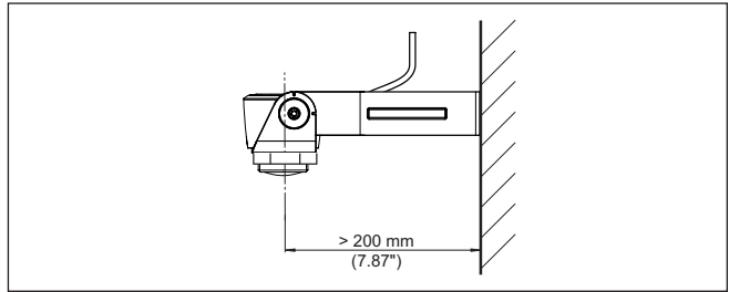
Fig. 6: Montage via een montagehoekstuk
