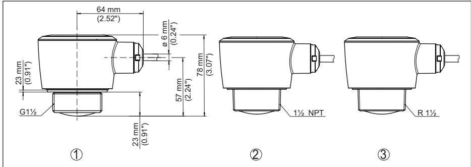
Fig. 29: Encombrement VEGAPULS C 22
