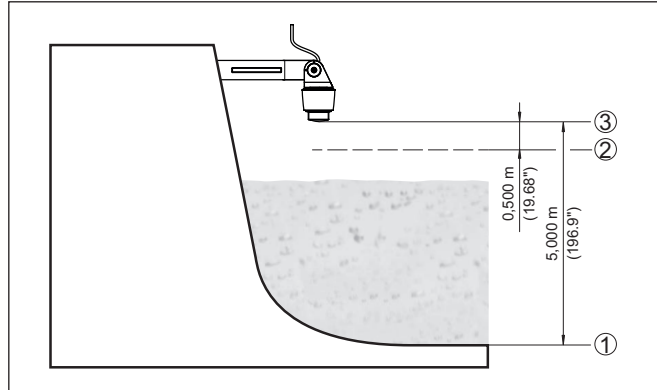
Fig. 25: Exemple de paramétrage réglage min./max.
