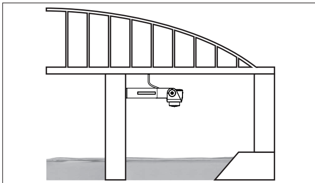
Fig. 15: Mesure de hauteur d'eau cours d'eau, Smontage du capteur sur un pilier de pont
