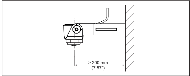
Fig. 6: Montage par une équerre de montage
