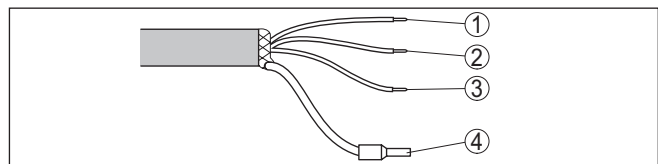
Fig. 20: Affectation des conducteurs du câble de raccordement raccordé de façon fixe
