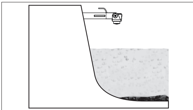
Fig. 16: Mesure de hauteur d'eau de barrage, montage du capteur sur une potence
