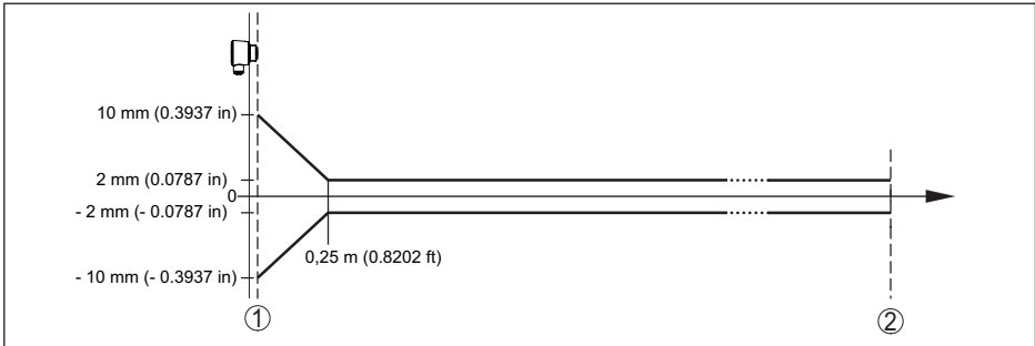
Fig. 28: Écart de mesure sous conditions de référence 10)
