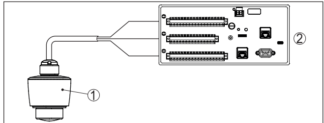
Fig. 4: Raccordement du VEGAPULS C 22 SDI-12 à l'enregistreur de données
