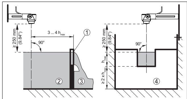
Fig. 18: Mesure du débit avec déversoir rectangulaire: h_{\text{max}} = remplissage max. du déversoir rectangulaire
