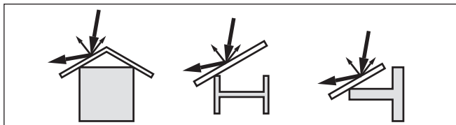
Rys. 14: Gładkie profile ostionić blachami rozpraszającymi
