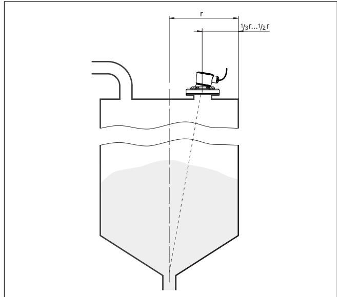
Rys. 16: Pozycja montażowa i ukierunkowanie
