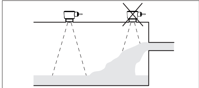
Rys. 11: Montaż sondy radarowej przy wpływającym medium
