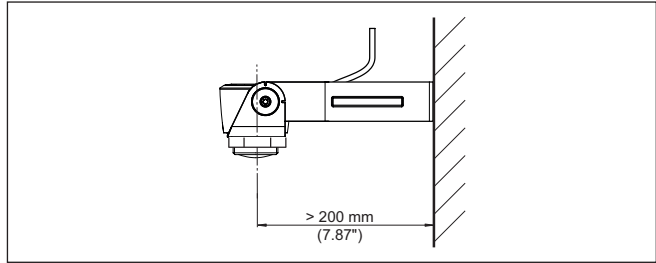
Rys. 6: Montaż za pomocą kątownika montażowego
