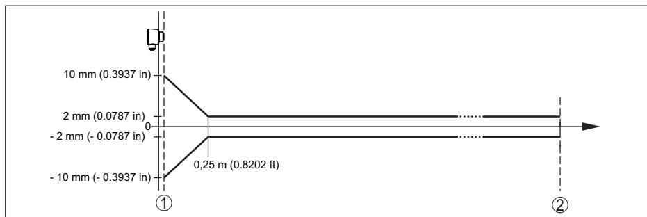
Rys. 32: Odchyłka pomiarowa w warunkach referencyjnych 10)
