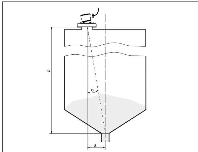
Rys. 17: Propozycja montażu z ukierunkowaniem VEGAPULS C 22
