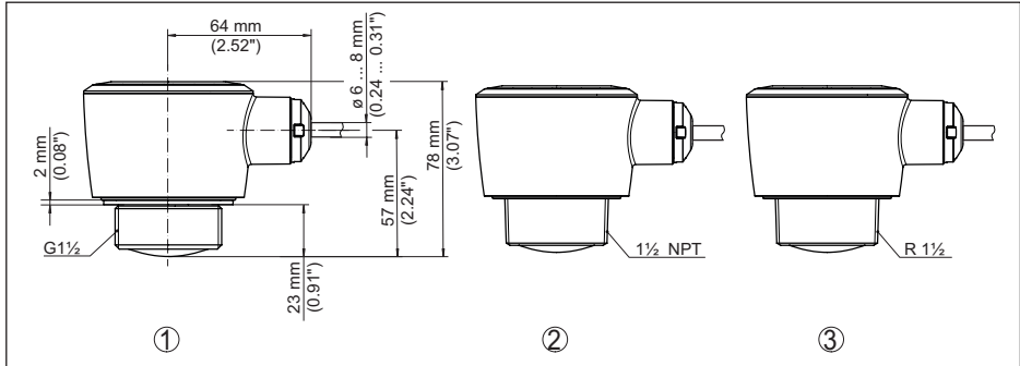
Rys. 33: Wymiary VEGAPULS C 22
