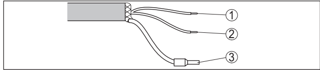
Rys. 21: Konfiguracja żył kabla trwale umocowanego do przyrządu
