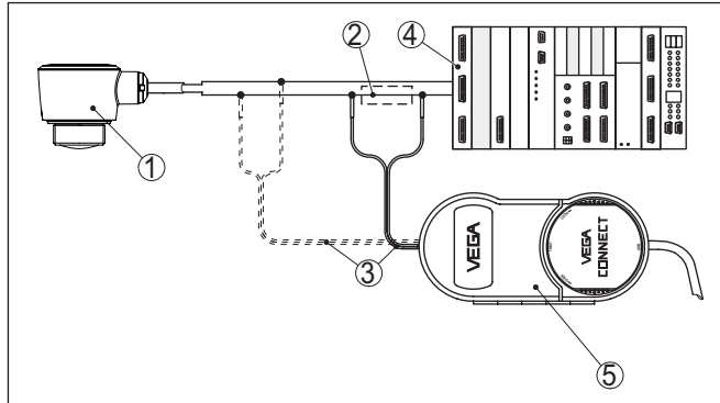
Rys. 26: Podłączenie PC do przewodu sygnałowego
