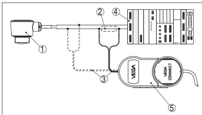
Rys. 4: Podłączenie PC do przewodu sygnałowego
