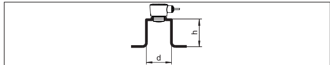
Rys. 13: Montaż króćca rurowego przy innych wymiarach króćca rurowego
