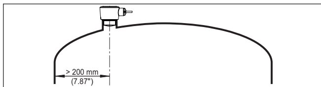
Rys. 8: Montaż sondy radarowej na okrągłym dnie zbiornika
