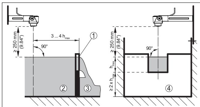
Rys. 19: Pomiar natężenia przepływu z przelewem prostokątnym: h_{max} = max. napełnienie przelewu prostokątnego
