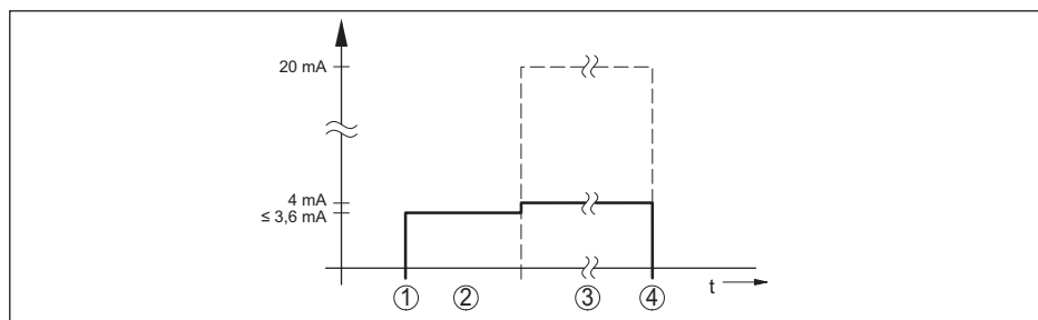
Rys. 31: Czas rozruchu i wysyłania wartości pomiarowych
