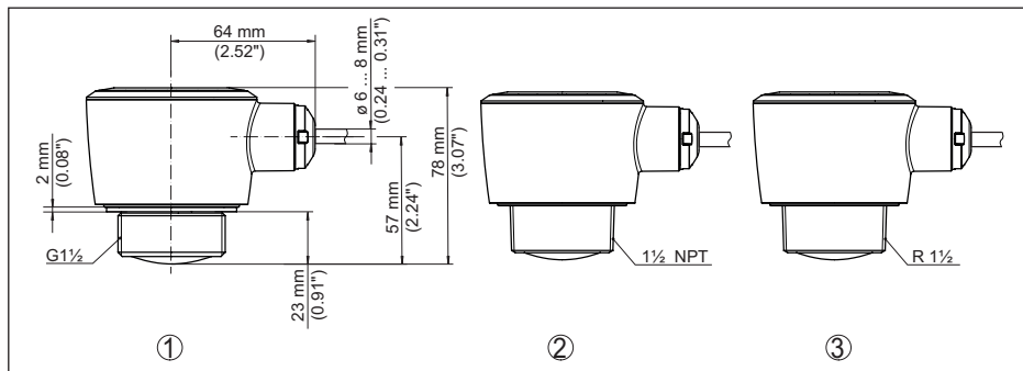
Fig. 33: Medidas VEGAPULS C 22
