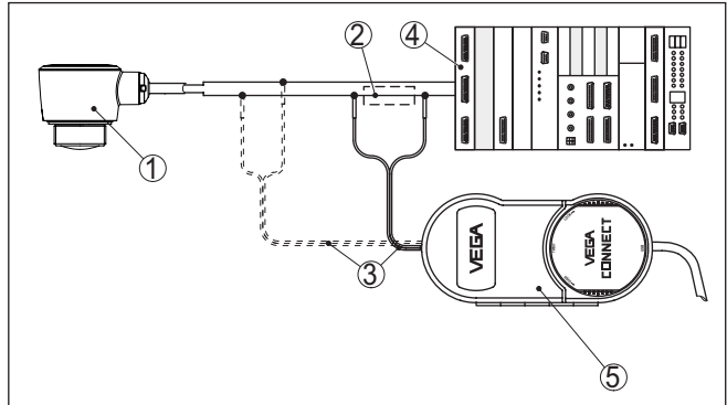
Fig. 26: Conexión del PC a la línea de señal
