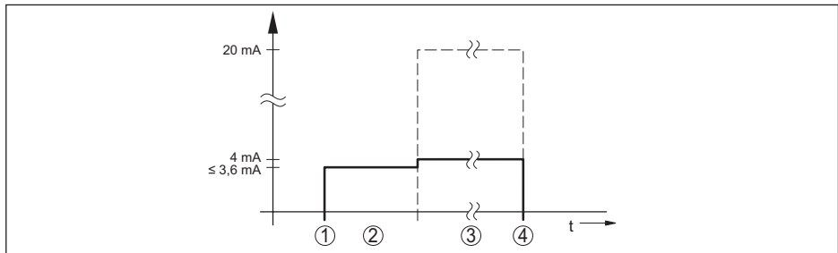
Fig. 31: Tiempo de aceleración y salida del valor de medición
