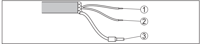
Fig. 21: Dotación de conductores, cable de conexión de conexión fija
