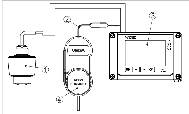
Fig. 27: Conexión del PC al controlador VEGAMET
