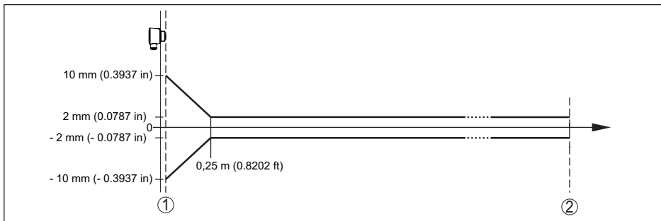
Fig. 32: Meetnauwkeurigheid onder referentiecondities 10)
