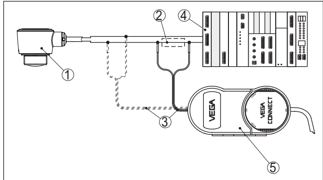
Fig. 26: Aansluiting van de PC op de signaalkabel
