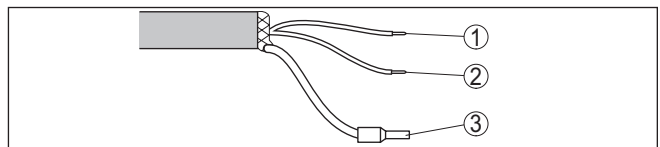
Fig. 21: Aderbezetting vast aangesloten aansluitkabel
