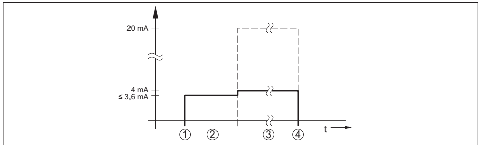
Fig. 31: Opstarttijd en uitsturen meetwaarde
