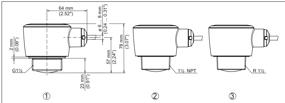
Fig. 33: Afmetingen VEGAPULS C 22
