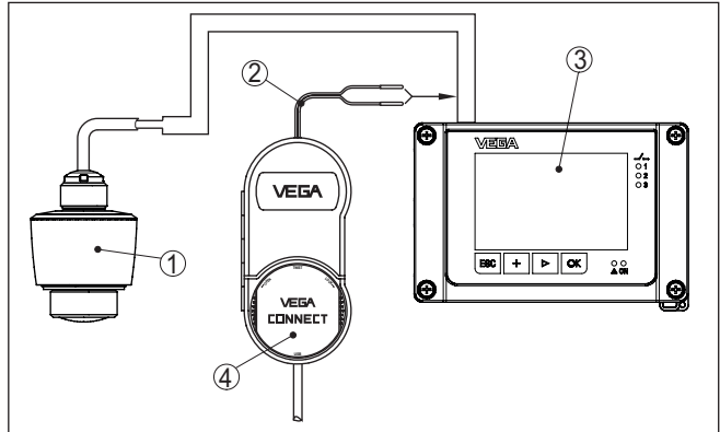
Fig. 27: Aansluiting van de PC op de regelaar VEGAMET
