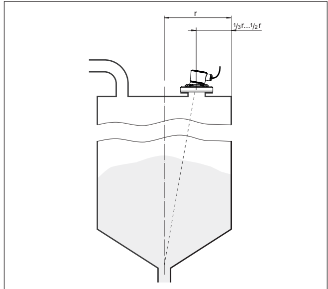
Fig. 16: Position de montage et orientation
