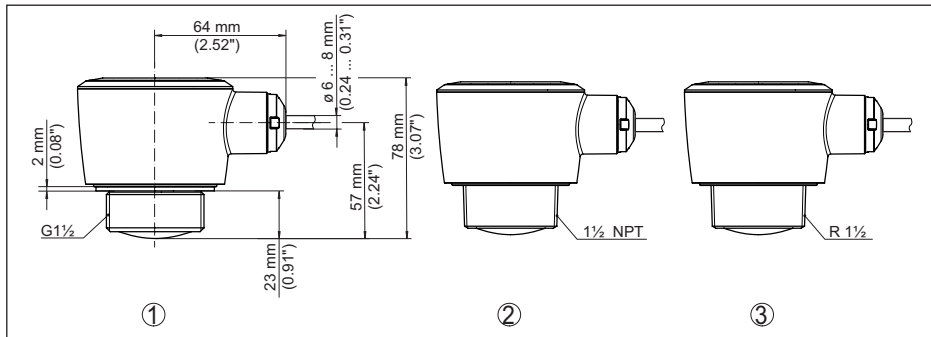
Fig. 33: Encombrement VEGAPULS C 22
