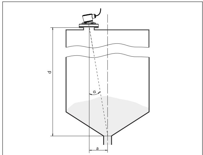
Fig. 17: Proposition pour un montage après orientation VEGAPULS C 22
