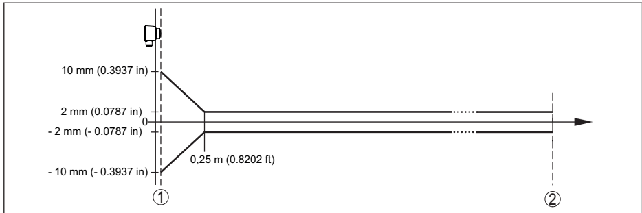
Fig. 32: Écart de mesure sous conditions de référence 10)
