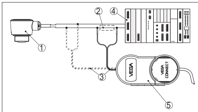
Fig. 26: Raccordement du PC à la ligne signal
