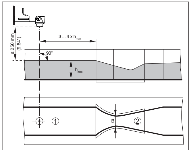
Fig. 20: Mesure du débit avec canal Venturi Khafagi : h_{max} = remplissage max. du canal ; B = resserrement max. du canal
