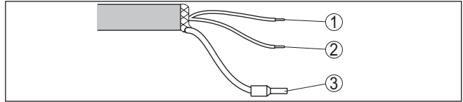
Fig. 21: Affectation des conducteurs du câble de raccordement raccordé de façon fixe
