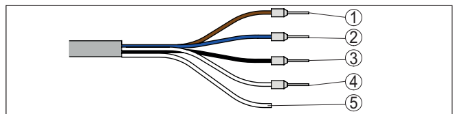
Fig. 20: Dotación de conductores, cable de conexión de conexión fija
