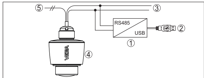
Fig. 25: Conexión del PC a la línea de señal
