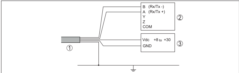
Fig. 30: Conexión del VEGAPULS C 21 a RTU Fisher ROC 809
