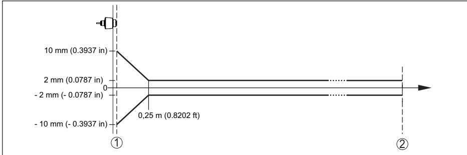
Fig. 29: Error de medición bajo condiciones de referencia 10)
