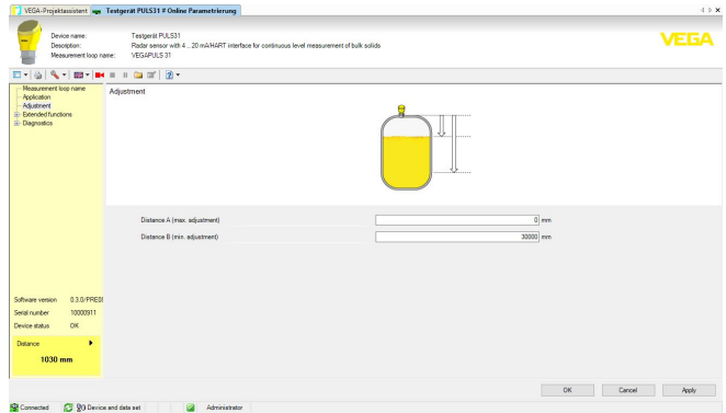
Fig. 26: Ejemplo de una vista DTM
