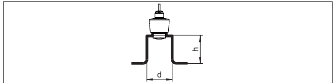
Fig. 12: Montaje de tubuladuras con medidas divergentes
