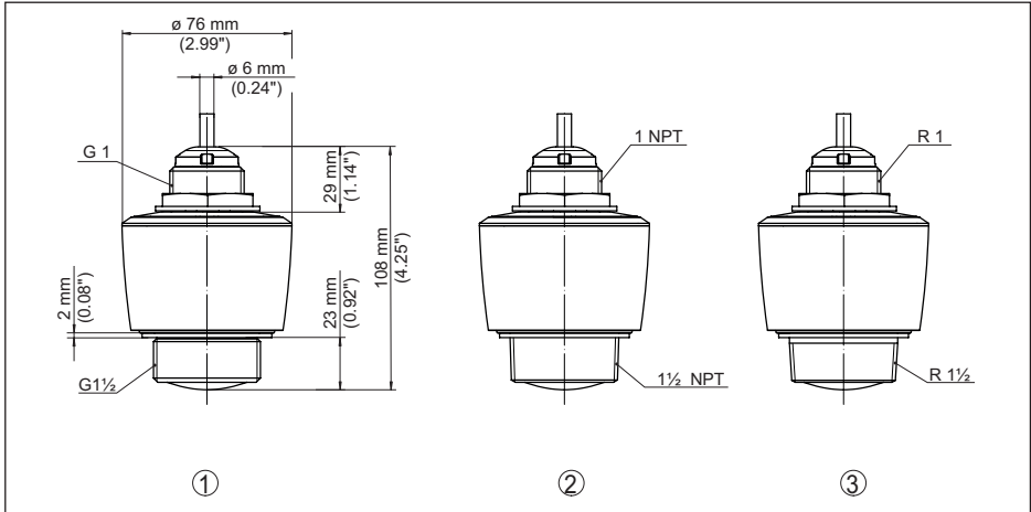
Fig. 31: Medidas VEGAPULS C 21
